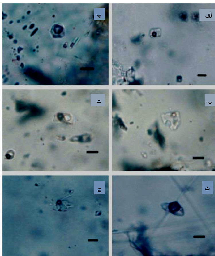
شکل ۵. شکل‌های مختلفی از میانبارهای شاری در کانی کوارتز کانسار باغو. باریک شدگی میانبار در شکل شماره ۵ - ج کاملاً مشخص است. مقیاس معادل ۱۰ um در نظر گرفته شد.
