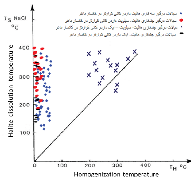
شکل ۸ نمودار دمای انحلال نمک در مقابل دمای همگن‌شدگی.
