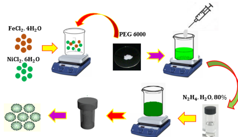
شکل ۲ فرآیند تهیه نانوذرات FeNi 3 به روش گرمایی.
