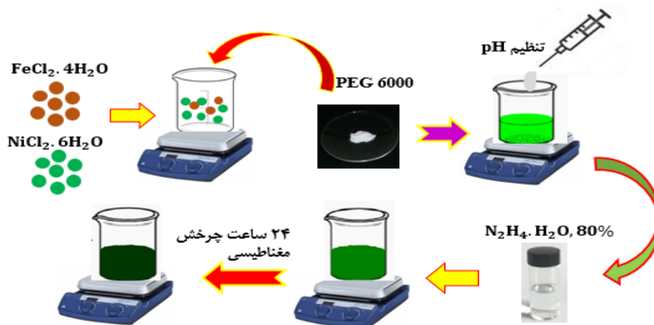
شکل ۳ فرآیند تهیه نانوذرات FeNi 3 به روش هم‌رسوبی.
