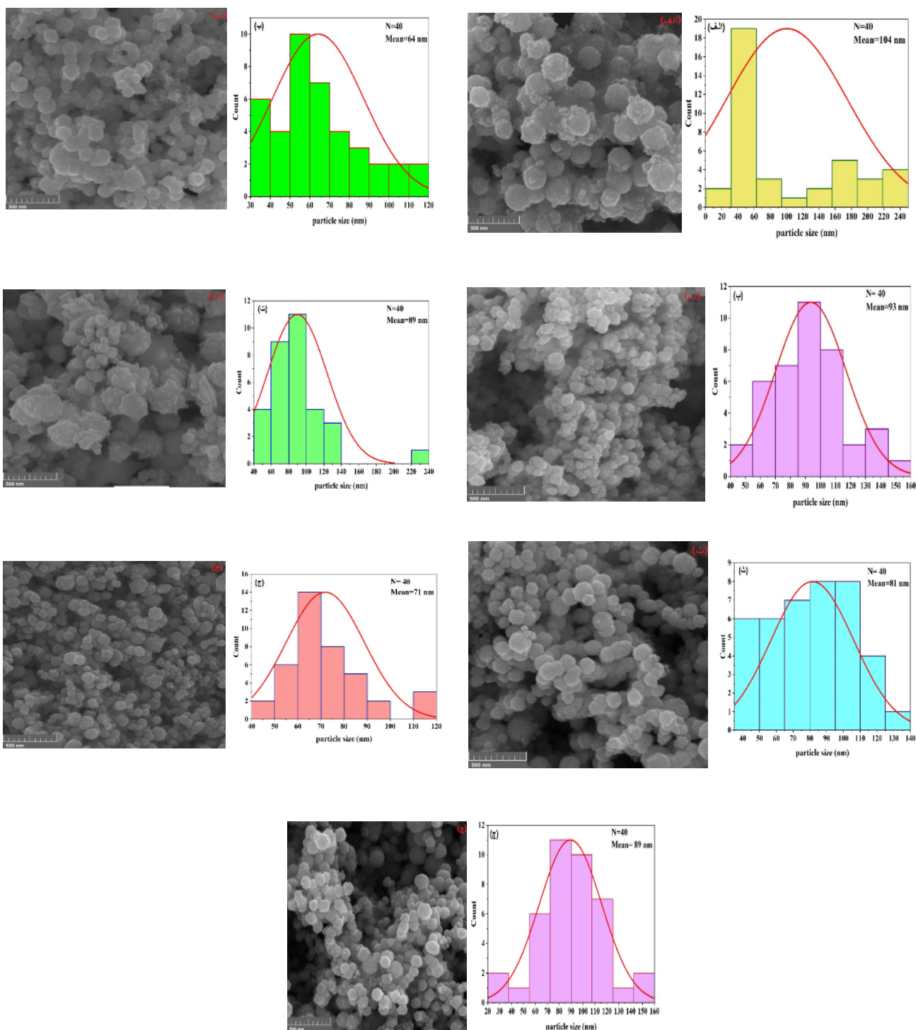
شکل ۵ تصاویر FESEM نانوذرات FeNi 3 تهیه شده به روش گرمایی با الف) ۵h-۱۰۰ °C، ب) ۱۰h-۱۰۰ °C، پ) ۱۵h-۱۰۰ °C (تصاویر الف، ب و پ با ۱ml هیدریت هیدرازین، ت) ۱۰h-۸۰ °C، ث) ۱۰h-۱۰۰ °C، ج) ۱۰h-۱۲۰ °C (تصاویر ت، ث و ج با ۳ml هیدریت هیدرازین و تهیه شده به چ) روش هم‌رسوبی.
