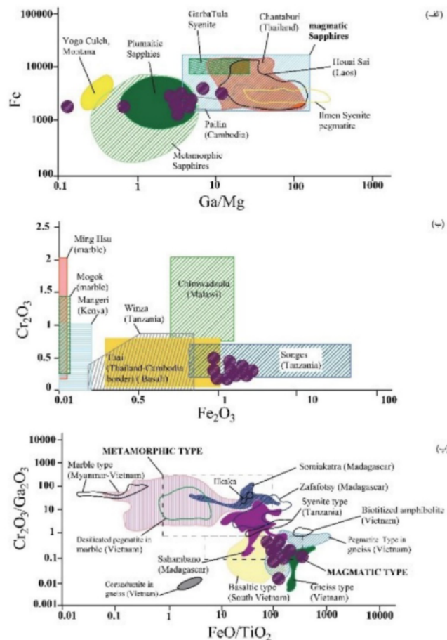
شکل ۶ نمودارهای رسم شده بر اساس داده‌های تجزیه شیمیایی بلورهای کروندوم خاکو به روش‌های XRF و ICP-MS: (الف) نمودار آهن (Fe) نسبت به Ga/Mg. نمودار پایه برگرفته از مراجع [۳۷، ۳۹، ۴۰] است، (ب) نمودار Cr 2 O 3 نسبت به Fe 2 O 3 که انواع ذخایر مختلف آفریقا را نشان می‌دهد. نمودار پایه برگرفته از مراجع [۲۲، ۳۶، ۴۱-۴۴] است.
