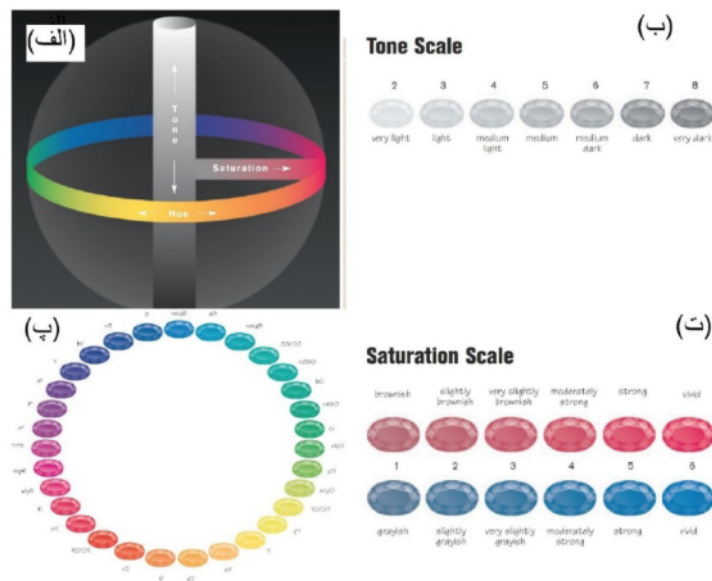
شکل ۷ (الف) مدل سه بعدی از عوامل اصلی ایجاد رنگ در اجسام جامد بلوری شفاف ارائه شده توسط موسسه گهرشناسی آمریکا (GIA). (ب). مقیاس عمق رنگ درباره دامنه تاریکی یک گوهر. سه استاندارد مهم عبارتند از ۳: روشن، ۵: متوسط و ۷: تاریک. (پ) نسبت نزدیکی به رنگ‌های اصلی یا رنگ مایه که ۳۱ رنگ گوهر به صورت استاندارد تعریف شده‌اند (استاندارد GIA). (ت). مقیاس اشباع.
