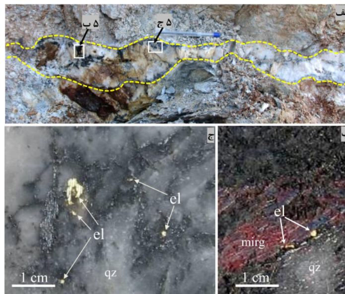
شکل ۵ تصویری از عدسی سیلیسی، که با خط چین زرد رنگ مشخص شده است و در بخش چینه‌سان کانسار رخداد دارد. در این عدسی سیلیسی، کانه‌های سولفوسالتی تیره رنگ تمرکز قابل توجهی دارند. ب و پ) ذرات الکتروم، در اندازه‌های ۰٫۵ تا ۴ میلی‌متر، در همراهی با کانه‌های سولفوسالتی مشاهده می‌شوند.
