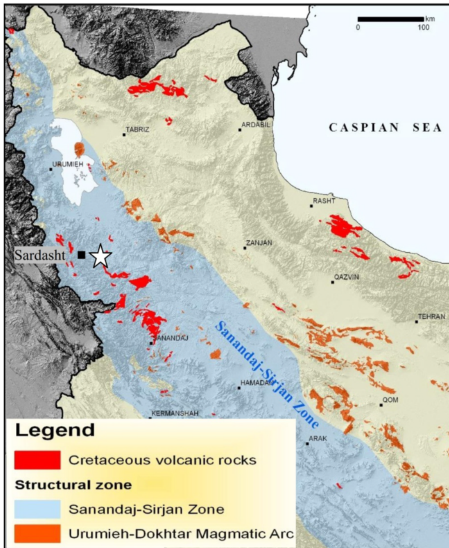
شکل ۱ موقعیت کانسار باریکا در پهنه سنندج-سیرجان. کانسار باریکا، که با ستاره سفید رنگ نشان داده شده است، در همراهی با سنگ‌های آتشفشانی (کرتاسه) رخ داده است.
