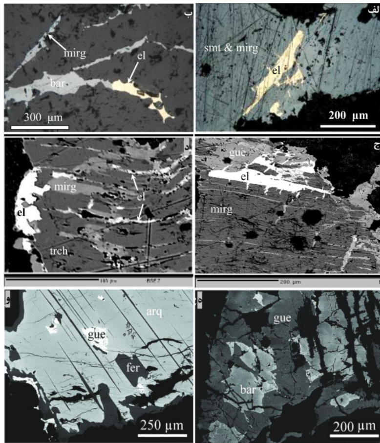
شکل ۶ تصاویر میکروسکوپ نوری بازتابی (الف، ب، ث، ج) و تصاویر میکروسکوپ الکترونی (BSE) (پ و ت) از رخداد برخی سولفوسالت‌ها و الکتروم در کانسنگ‌های طلا دار باریکا: (الف) الکتروم در همراهی با اسمایتیت و میرارژیریت، (ب) الکتروم در همراهی با باریکائیت و میرارژیریت، (پ) الکتروم در همراهی با گتاردیت و میرارژیریت، (ت) الکتروم در همراهی با میرارژیریت و تریچمانیت، (ث) باریکائیت، به‌طور قابل توجهی توسط گتاردیت جانشین شده است. (ج) گتاردیت و فردوسی‌ایت به‌طور قابل توجهی توسط آرسن کواتراندوریت جانشین شده‌اند. arq: آرسن کواتراندوریت، bar: باریکائیت، el: الکتروم، fer: فردوسی‌ایت، mirg: میرارژیریت، smit: اسمایتیت، trch: تریچمانیت و gue: گتاردیت).
