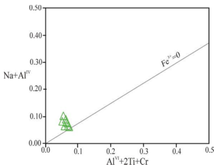
شکل ۱۲ برآورد مقدار گریزندگی اکسیژن در محیط تشکیل گدازه‌های آندزیتی منطقه زولسک براساس ترکیب شیمیایی کلینوپیروکسن‌ها [۴۵].
