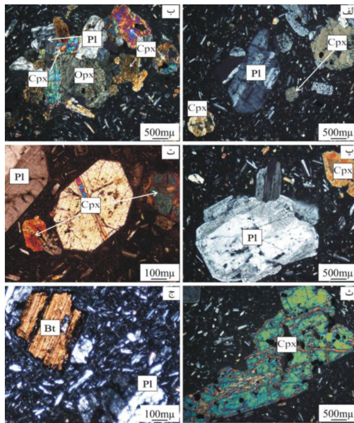
شکل ۲ ویژگی‌های میکروسکوپی آندزیت‌های منطقه زولسک: الف) بافت پورفیری با خمیره میکرولیتی شیشه‌ای، ب) بافت گلوپورفیری و حضور کانی‌های پلاژیوکلاز، کلینوپیروکسن و ارتوپیروکسن، پ) درشت بلورهای پلاژیوکلاز دارای منطقه‌بندی و بافت غربالی در حاشیه، ت) کلینوپیروکسن شکل‌دار، ث) کلینوپیروکسن بی‌شکل و دارای حاشیه خلیجی و ج) درشت بلور بیوتیت (همه شکل‌ها در نور قطبیده متقاطع، XPL ثبت شده‌اند) نشانه‌های اختصاری کانی‌ها برگرفته از مرجع [۲۶] هستند.
