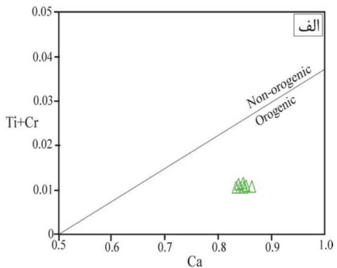
شکل ۸ الف) نمودار Ti+Cr نسبت به Ca [۱۴] و ب) نمودار F1 نسبت به F2 [۱۳] برای تعیین محیط زمین ساختی گدازه‌های آندزیتی منطقه زولسک بر اساس ترکیب کلینوپیروکسن: (OFB): بازالت‌های بستر اقیانوس، (WPT): بازالت‌های تولئیتی میان صفحه‌ای، (WPA): بازالت‌های قلیایی میان صفحه‌ای و (VAB): بازالت‌های کمان آتشفشان).
