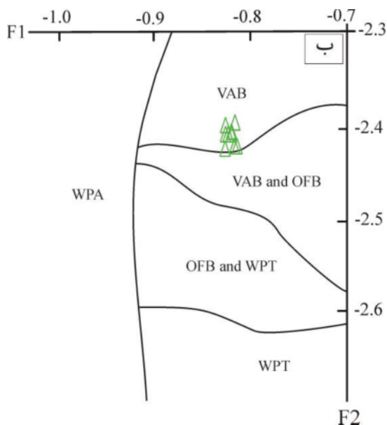
شکل ۸ الف) نمودار Ti+Cr نسبت به Ca [۱۴] و ب) نمودار F1 نسبت به F2 [۱۳] برای تعیین محیط زمین ساختی گدازه‌های آندزیتی منطقه زولسک بر اساس ترکیب کلینوپیروکسن: (OFB): بازالت‌های بستر اقیانوس، (WPT): بازالت‌های تولئیتی میان صفحه‌ای، (WPA): بازالت‌های قلیایی میان صفحه‌ای و (VAB): بازالت‌های کمان آتشفشان).
