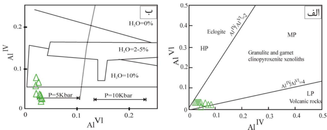
شکل ۱۳ موقعیت کلینوپیروکسن‌ها در نمودارهای توزیع آلومینیم در جایگاه‌های چهاروجهی و هشت‌وجهی؛ الف) برای برآورد فشار [۴۷] و ب) تعیین درصد آب ماگما [۴۸].
