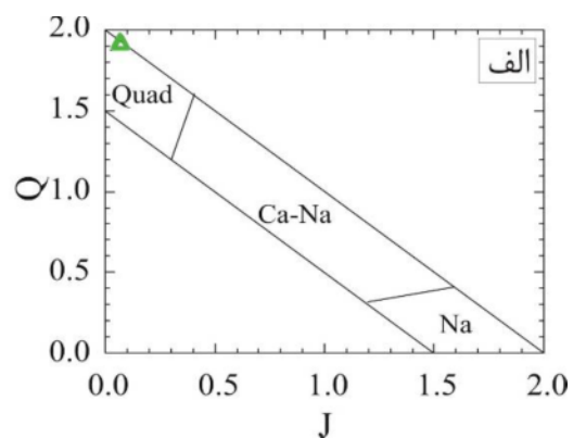
شکل ۵ الف) موقعیت کالینوپيروكسن‌ها و ب) ارتوپيروكسن‌های منطقه زولسک در نمودار Q-J [۳۴، ۳۵] ( Q = Ca + Mg + Fe + 2Na و J = 2Na ).
