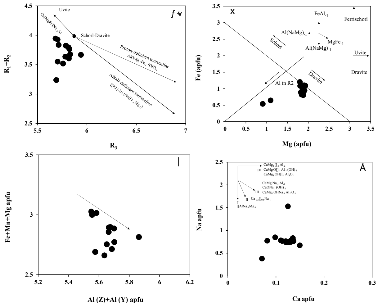
شکل ۵ الف) نمودار R_1+R_2 نسبت به R_3 [۲۰]؛ R_3 (Al+Ti)؛ R_2=Ca+Na ؛ R_1=Fe+Mn+Mg ؛ ب) نمودار Fe نسبت به Mg [۱۵]؛ پ) ارتباط منفی بین Al^t و Fe+Mg+Mn ؛ ت) در آن نمودار Ca نسبت به Na و جایگاه نمونه‌ها.
