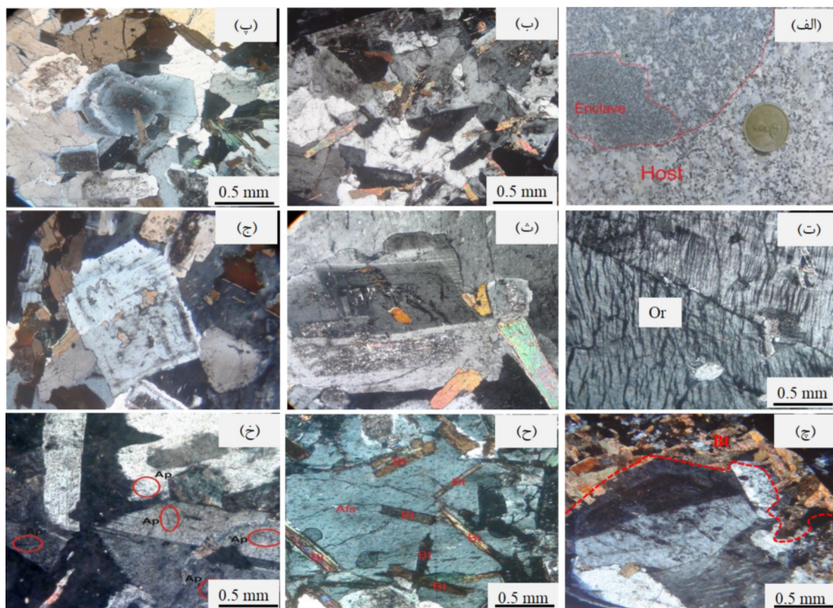
شکل ۲ تصاویر صحرائی و میکروسکوپی از توده گرانیتوئیدی گوشه: الف) برونوم‌های ریزدانه‌ای بیضوی شکل و زاویه‌دار، ب) کانی‌های موجود در واحد گرانودیوریتی، پ) منطقه بندی، انحلال و خورده شدگی پلاژیوکلاز در واحد مونوزگرانیتی (در نور قطبیده متقاطع، XPL)، ت) بافت پرتیت در ارتوز (در نور XPL)، ث) لبه انحلالی در پلاژیوکلاز (در نور XPL)، ج) میانبر کانی‌های بیوتیت، کوارتز و پلاژیوکلاز در فلدسپارهای قلیایی (پرتیت) و تشکیل بافت خال‌خال (در نور XPL)، چ) انباشت لخته‌های مافیک بیوتیت و کانی‌های کدر (در نور XPL)، ح) بیوتیت‌های تیغه‌ای در درشت بلور فلدسپار (در نور XPL) و خ) آپاتیت‌های سوزنی در پلاژیوکلازها (در نور XPL). نشانه‌های اختصاری کانی‌ها (Ap): آپاتیت، Qtz: کوارتز، Afs: فلدسپار قلیایی، Bi: بیوتیت و Or: ارتوکلاز) برگرفته از مرجع [۳۱] است.
