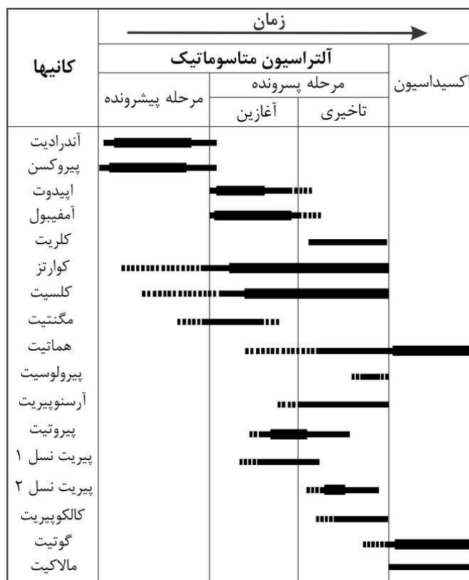
شکل ۶ توالی همبری کانی‌ها در نهشته معدنی سنجدک III، بخش شرقی معدن سنگ آهن سنگان.
