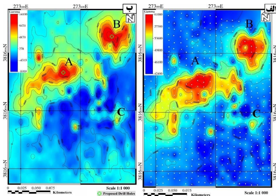
شکل ۸ الف) نقشه مغناطیس کل (TMI) همراه با نمایش جایگاه ایستگاه‌های برداشت شبکه مغناطیس‌سنجی زمینی، منطقه سنجک III، ب) نقشه انتقال یافته به قطب (RTP) به همراه نقاط حفاری پیشنهادی در مرکز ناهنجاری‌های زمین مغناطیسی A و B.
