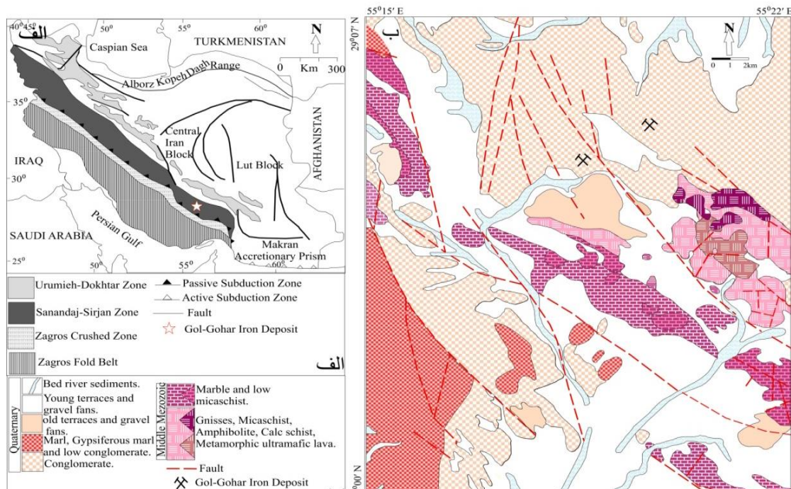
شکل ۱ الف) موقعیت منطقه گل‌گهر بر پهنه ساختاری سنندج-سیرجان و جایگاه این پهنه نسبت به دیگر پهنه‌های ساختاری در ایران [۹-۱۱]؛ ب) نقشه زمین‌شناسی منطقه گل‌گهر و موقعیت کانسار آهن گل‌گهر بر آن [۱۲].
