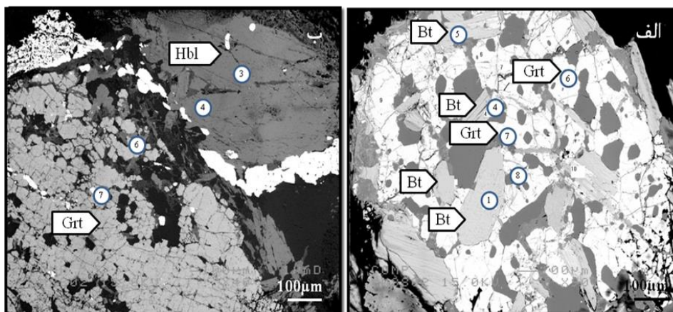
شکل ۶ نقاط تجزیه شده توسط تجزیه ریزکاو الکترونی که نشان دهنده الف) وجود بیوتیت درون گارنت‌های متاپلیتی‌ها و ب) همجواری هورنبلند و گارنت در گارنت آمفیبولیت‌های منطقه گل‌گهر هستند.
