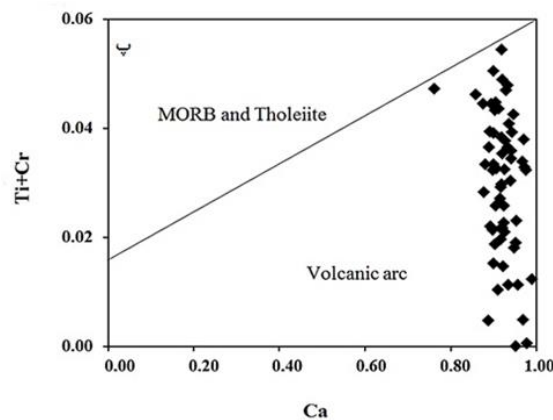
شکل ۹ نمودارهای تعیین سری ماگمایی و تعیین محیط زمین ساختی، سنگ‌های دیابازی منطقه ده ظهیر الف) نمودار تغییرات درصد وزنی Al_2O_3 نسبت به درصد وزنی SiO_2 در کانی کلینوپیروکسن [۱۹]، ب) نمودار تغییرات درصد وزنی Al_2O_3 نسبت به درصد وزنی TiO_2 [۱۸]، و پ) نمودار مقدار Ca نسبت به Ti+Cr در کانی کلینوپیروکسن [۱۹].
