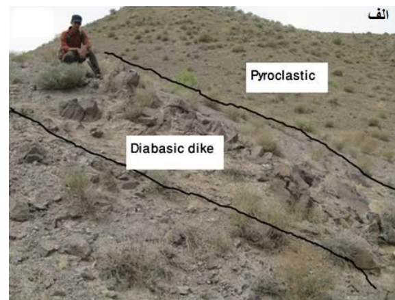
شکل ۲ الف) نفوذ دایک دیابازی در سنگ‌های آذرآواری منطقه ده‌ظهر و ب) نفوذ توده دیابازی به درون گدازه‌های آندزیتی.
