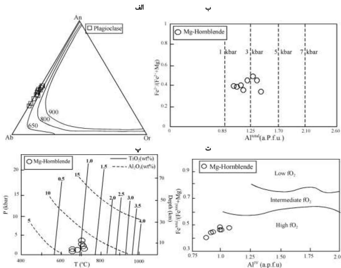
شکل ۵ الف- نمودار آنورتیت-آلبیت-ارتوکلاز به منظور دماسنجی کانی‌های فلدسپار موجود در توده گرانیتی اسماعیل آباد در فشار ۱ کیلو بار [۱۶]. ب- نمودار فشارسنجی آمفیبول‌های موجود در این گرانیت‌ها [۱۷]. پ- نمودار تغییرات دما-فشار-عمق بر اساس مقدار \text{TiO}_2 و \text{Al}_2\text{O}_3 موجود در آمفیبول‌ها [۱۸]. ت- بررسی گریزندگی اکسیژن ماگمای مولد گرانیت‌های مورد بررسی براساس ترکیب آمفیبول‌ها [۱۹].
