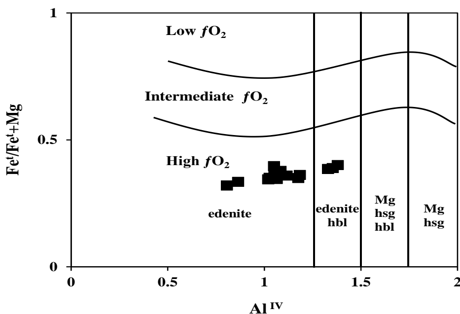
شکل ۸ نمودار گریزندگی اکسیژن بر پایه ترکیب آمفیبول [۴] که بالا بودن گریزندگی اکسیژن در زمان تبلور آمفیبول‌های گرانیتوئید جبال بارز را نشان می‌دهد.
