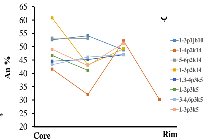
شکل ۵ الف) رده‌بندی پلاژیوکلازها در گرانیتوئید جبال بارز. ب) الگوی منطقه‌بندی بلورهای پلاژیوکلاز از مرکز به لبه در گرانیتوئید جبال بارز.
