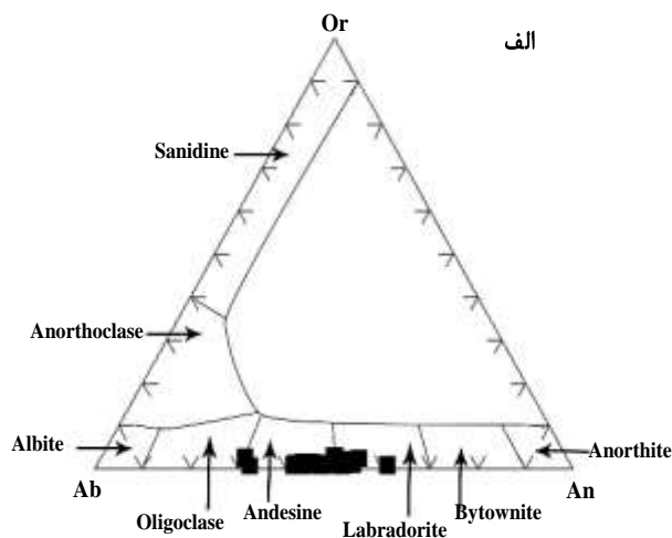
شکل ۵ الف) رده‌بندی پلاژیوکلازها در گرانیتوئید جبال بارز. ب) الگوی منطقه‌بندی بلورهای پلاژیوکلاز از مرکز به لبه در گرانیتوئید جبال بارز.
