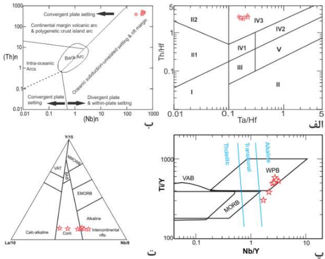
شکل ۸ نمودارهای تشخیص محیط زمین‌ساختی سنگ‌های آتشفشانی منطقه سیارده: نمونه‌های منطقه در نمودار (الف) [۴۴]، در گستره بازالت‌های مناطق کمربندهای کشتی درون قاره‌ای یا کافت اولیه، در نمودار (ب) [۴۵]، در گستره محیط‌های واگرای کافتی درون صفحه، در نمودار (پ) [۴۶]، در گستره بازالت‌های درون صفحه‌ای و در گستره قلیایی، و در نمودار (ت) [۴۷]، در گستره ماگماهای قلیایی کافت‌های درون قاره‌ای واقع شده‌اند. (علائم اختصاری شکل الف: I = منطقه N-MORB در کناره صفحات واگرا، II = بازالت‌های لبه صفحات همگرا، III = بازالت‌های کمان اقیانوسی، II2 = بازالت‌های کرانه قاره‌ای، III = مناطق MORB - نوع E و MORB نوع T و بازالت‌های جزایر اقیانوسی درون صفحه اقیانوسی، IV = بازالت‌های درون صفحه‌ای قاره‌ای، IV1 = کافت‌های درون قاره‌ای + تولیت‌های کافت‌های کرانه‌ی قاره، IV2 = بازالت‌های قلیایی کافت‌های درون قاره‌ای، IV3 = بازالت‌های مناطق کمربندهای کشتی درون قاره‌ای یا کافت اولیه، V = بازالت‌های زبانه‌های مناطق گوشته‌ای؛ شکل پ) MORB: بازالت‌های پشته میان اقیانوسی؛ VAB بازالت‌های کمان آتشفشانی؛ WPB بازالت‌های درون صفحه‌ای؛ شکل ت) BAB: بازالت‌های پشت کمان آتشفشانی؛ EMORB: بازالت‌های غنی‌شده پشته میان اقیانوسی؛ NMORB: بازالت‌های عادی پشته میان اقیانوسی و VAT: تولیت‌های کمان آتشفشانی)
