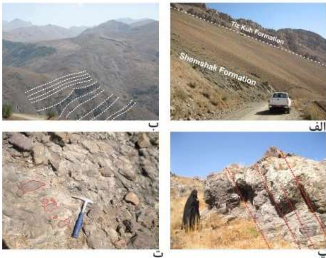
شکل ۲ تصاویر صحرایی برخی از رخنمون‌های منطقه مورد بررسی: الف) قرارگیری سازند تیزکوه بر سازند شمشک؛ ب) روانه‌های چینه‌سان منطقه سپارده؛ پ) درزه‌های انقباضی در یکی از روانه‌ها؛ ت) برش آتشفشانی شیشه‌آواری شامل قطعات گرد مافیک در زمینه فلسیک.
