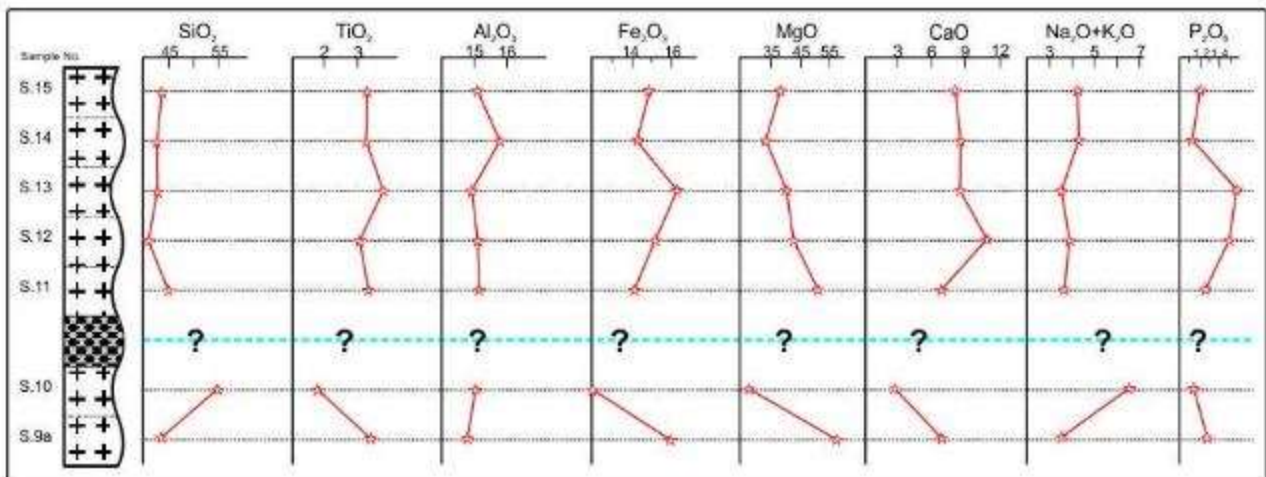
شکل ۶ نمودار تغییر مقادیر اکسیدهای عناصر اصلی در توالی نمونه‌های برداشت شده (بدون مقیاس). علامت ؟ مربوط به نمونه آب‌آوری (شکل ۲-ت) است.
