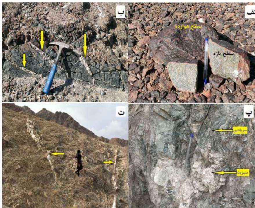
شکل ۳ الف) سطح تازه و هوازده در سنگ‌های فرامافیک منطقه. ب) تأثیر فشارهای زمین‌ساختی در خورد شدن سنگ‌ها و تشکیل رگه‌های کربناته در بین لایه‌های آن. پ) سریانتینی شدن و تشکیل منیزیت. ت) رگه‌های سفیدرنگ مربوط به کربنات‌های ثانویه در سنگ‌های فرامافیک نازدشت [۶].
