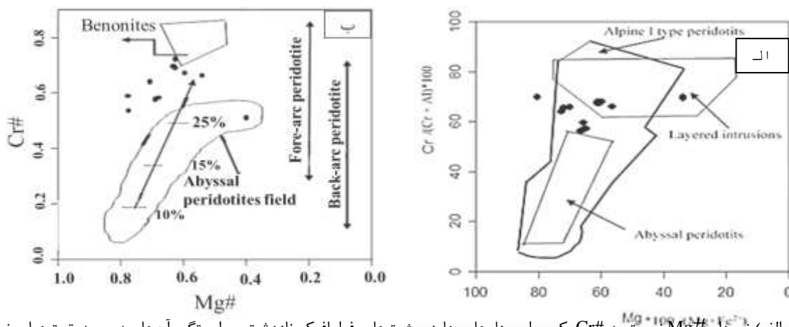
شکل ۱۲ (الف) نمودار Cr\# نسبت به Mg\# کروم اسپینل‌های هارزبورژیت‌های فرامافیک نازدشت و وابستگی آن‌ها به پریدوتیت‌های نوع آلپی [۱۱]. (ب) نمونه هارزبورژیت‌های فرامافیک نازدشت در نمودار Cr\# نسبت به Mg\# اسپینل‌های آن. گستره‌ی آبیسال، جلوی قوس و پشت قوس به ترتیب از مراجع [۳۲، ۳۱، ۱۳] و گستره بونینیت از مرجع [۱۱] آورده شده‌اند. نماد علامت‌دار شده نشان دهنده درصد ذوب سنگ پریدوتیت میزبان بر اساس محاسبات مرجع [۳۰] است.
