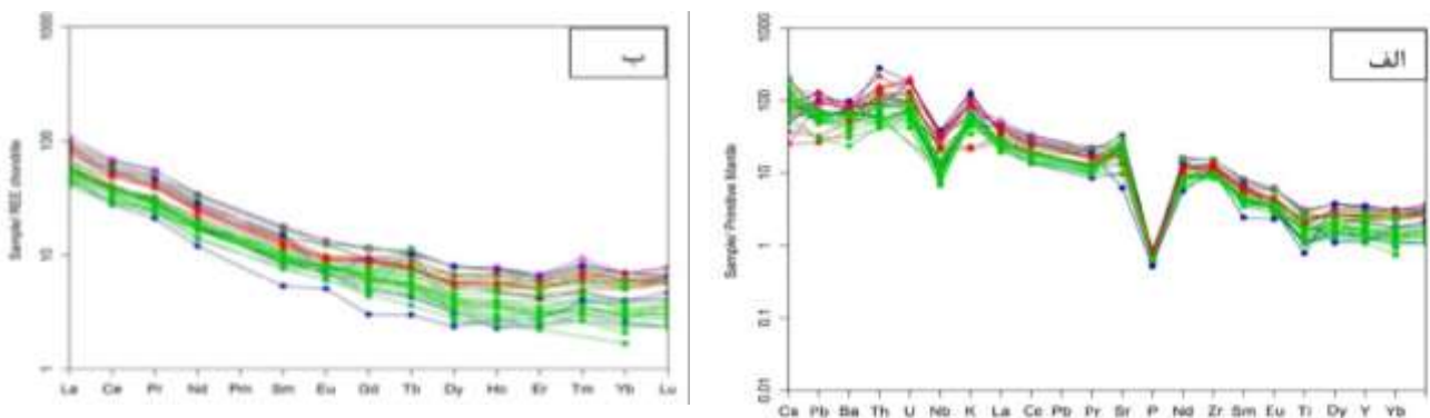
شکل ۶ نمودارهای چند عنصری برای نمونه‌های آداکیتی موجود در نوار ماگمایی قوچان-اسفراین، الف) بهنجار شده به گوشته اولیه [۴۳] و ب) بهنجار به کندریت [۴۴].
