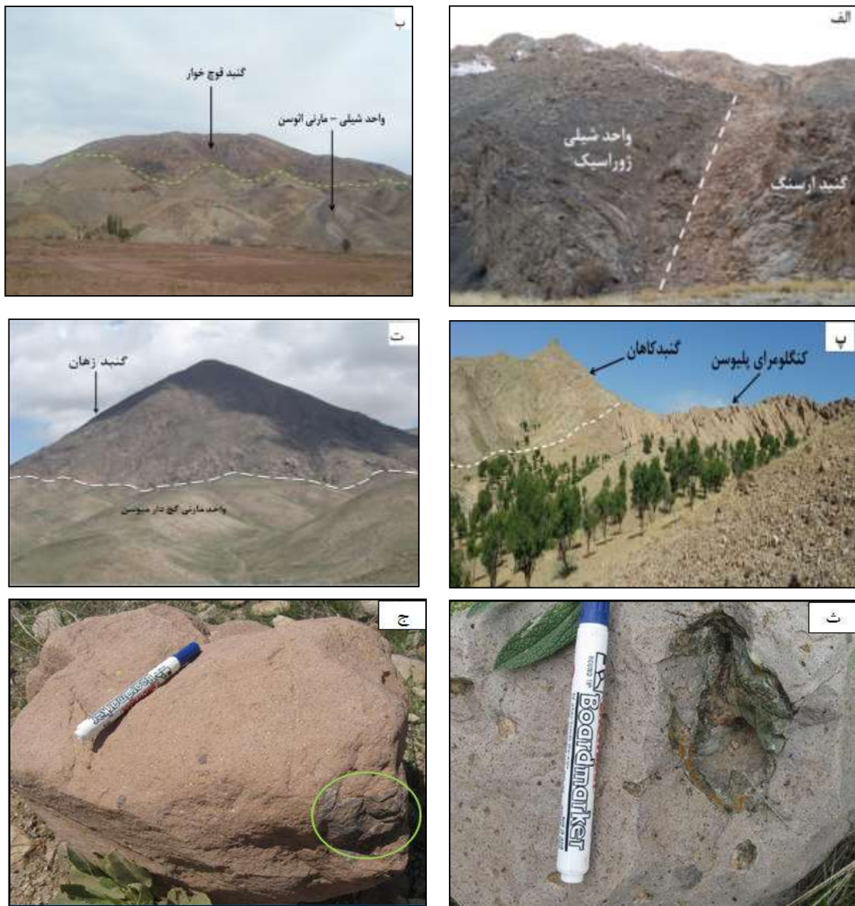
شکل ۲ الف، ب، پ، ت) تصاویر صحرایی از رخنمون‌های گنبد‌های آداکیتی نوار ماگمایی قوچان- اسفراین در واحدهای مختلف رسوبی منطقه، ت و ج) حضور درونبوم‌های واحد شیلی - مازنی ائوسن در سنگ‌های داسیتی مارکوه (جنوب روستای ینگجه).
