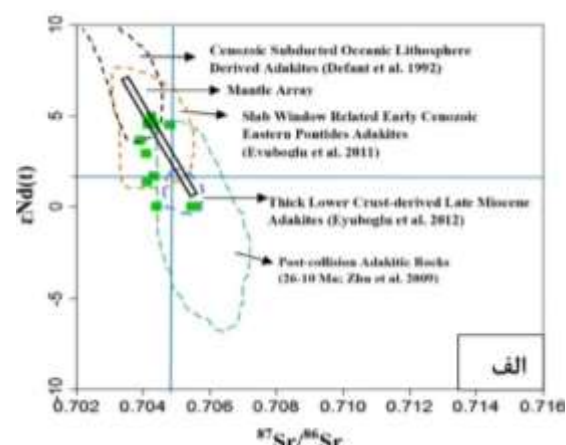
شکل ۹ الف) نمودار ^{87}\text{Sr}/^{86}\text{Sr} آغازین نسبت به \epsilon\text{Nd}(t) برای سنگ‌های آداکیتی نئوزن در نوار ماگمایی قوچان-اسفراین [۵۲]، ب) نمودار تغییرات ^{87}\text{Sr}/^{86}\text{Sr} نسبت به Rb [۵۷].
