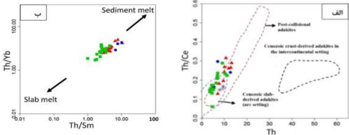
شکل ۱۲ الف) نمودار تغییرات Th نسبت به Th/Ce که میدان‌های مشخص شده بر نمودار برگرفته از مرجع [۶۶] است، ب) نمودار تغییرات Th/Yb نسبت به Th/Sm برای سنگ‌های آداکیتی نتوزن در منطقه مورد بررسی که نشان دهنده روند خطی و قرارگیری نمونه‌ها در بین گدازه‌های برآمده از ذوب ورقه فرورنده و رسوبات است، موقعیت گدازه تختال برگرفته از مرجع [۴۳].
