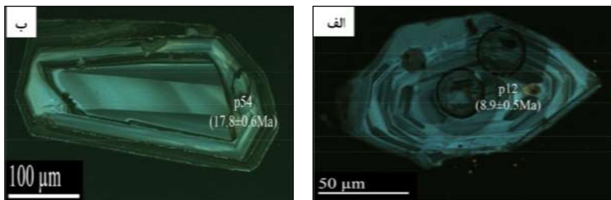
شکل ۷ تصاویر کاند تابناکی (CL) تهیه شده از نمونه‌های زیرکن جدا شده از دو نمونه، الف) داسیتی (Shykh1) و ب) تراکی آندزیتی (AR4) گنبد‌های آداکیتی نوار ماگمایی قوچان - اسفراین.
