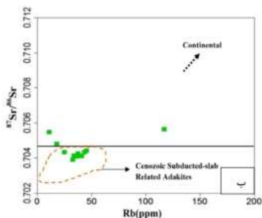
شکل ۹ الف) نمودار ^{87}\text{Sr}/^{86}\text{Sr} آغازین نسبت به \epsilon\text{Nd}(t) برای سنگ‌های آداکیتی نئوزن در نوار ماگمایی قوچان-اسفراین [۵۲]، ب) نمودار تغییرات ^{87}\text{Sr}/^{86}\text{Sr} نسبت به Rb [۵۷].
