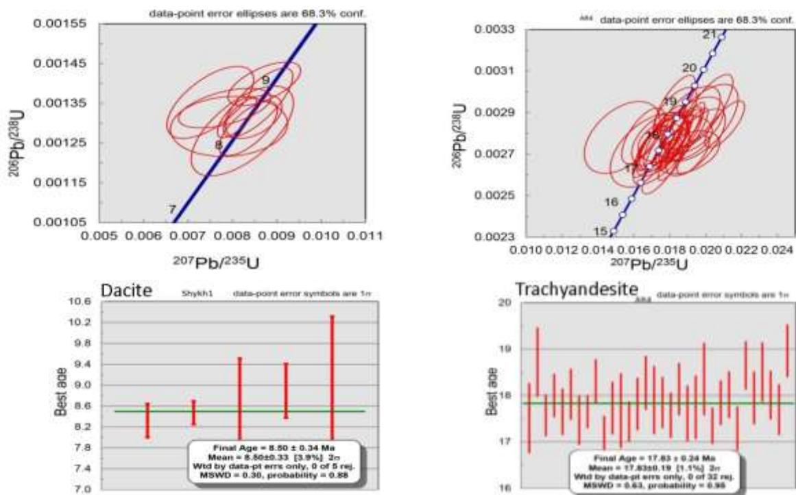
شکل ۸. نمودارهای تعیین سن سازگاری و میانگین سن بر اساس نتایج تجزیه‌های ایزوتوپی U-Pb بر زیرکن جدا شده از نمونه‌های داسیتی (Shykh1) و تراکی آندزیتی (AR4) گنبدی‌های آداکیتی نوار ماگمایی قوچان - اسفراین.
