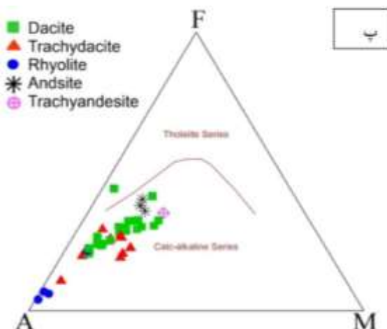
شکل ۴ الف) موقعیت قرارگیری نمونه‌های سنگی بر نمودار SiO_2 نسبت به مجموع قلیایی‌ها (Na_2O + K_2O) [۳۷]، ب) نمودار K_2O نسبت به SiO_2 [۳۸]، پ) نمودار AFM و موقعیت نمونه‌ها در گستره سنگ‌های آهکی-قلیایی [۳۹]، ت) نمودار A/CNK نسبت به A/NK که نشان دهنده ماهیت مت‌آلومین تا پرآلومین نمونه‌های مورد بررسی است [۴۰].
