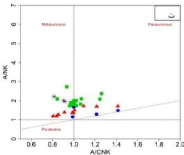
شکل ۴ الف) موقعیت قرارگیری نمونه‌های سنگی بر نمودار SiO_2 نسبت به مجموع قلیایی‌ها (Na_2O + K_2O) [۳۷]، ب) نمودار K_2O نسبت به SiO_2 [۳۸]، پ) نمودار AFM و موقعیت نمونه‌ها در گستره سنگ‌های آهکی-قلیایی [۳۹]، ت) نمودار A/CNK نسبت به A/NK که نشان دهنده ماهیت مت‌آلومین تا پرآلومین نمونه‌های مورد بررسی است [۴۰].
