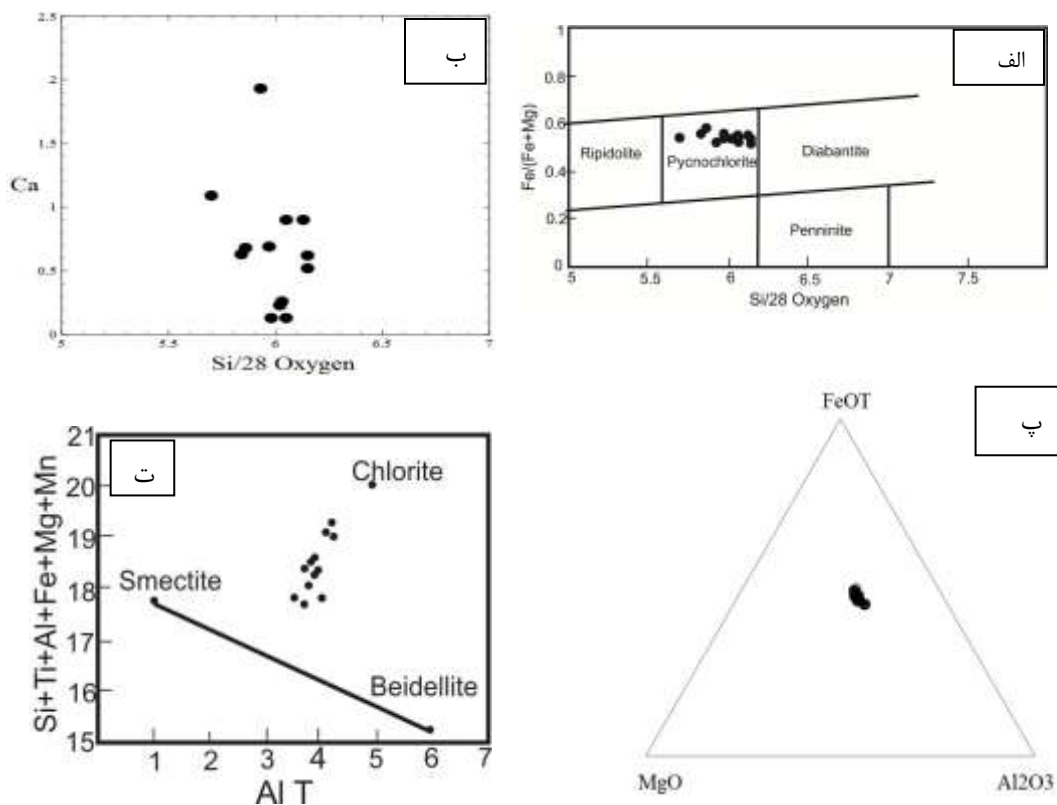
شکل ۴ نمونه‌های مورد بررسی بر الف) نمودار رده‌بندی کلریت‌ها [۱۳] و ب) نمودار Ca-Si، پ- نمونه کلریت‌های مورد بررسی بر نمودار MgO-FeO-Al 2 O 3 ، ت) گستره ترکیبی کلریت‌های مورد بررسی [۳۰]، این کلریت‌ها دارای لایه‌هایی از کانی‌های اسمکتیت هستند.
