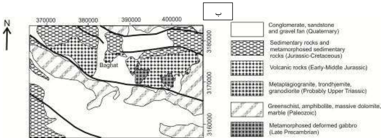
شکل ۱ الف- موقعیت منطقه مورد بررسی بر نقشه ایران. ب- نقشه ساده شده زمین شناسی باغات (۱:۱۰۰۰۰۰) [۸].
