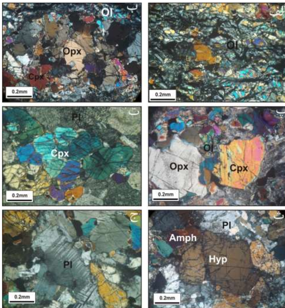
شکل ۳ الف- فراوانی کانی الیوین برشی شده و ب- بلورهای ارتوپیروکسن و کلینوپیروکسن در فرامافیک‌های لایه‌ای (لرزولیت پلاژیوکلازدار)، پ- کانی‌های پیروکسن و الیوین با بافت‌های انباشتی به همراه پلاژیوکلاز سوسوریتی شده، ت- بلورهای کلینوپیروکسن به همراه پلاژیوکلاز با بافت انباشتی در الیوین گابروها، ث- بلورهای هیپرستن، آمفیبول و پلاژیوکلاز انباشتی و ج- بلورهای پلاژیوکلاز با بافت انباشتی بین دانه‌هایی از پیروکسن در گابرونوریت‌ها. گفتنی است که همه عکس‌ها در نور قطبیده متقاطع تهیه شده‌اند.
