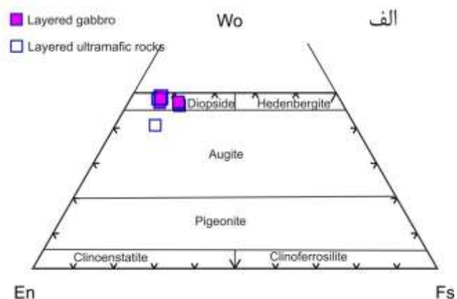
شکل ۴ موقعیت کلینوپیروکسن‌های گابروهای لایه‌ای جنوب ارزوتیه الف- در نمودار En-Fs-Wo [۱۶] و ب- در نمودار J-Q [۱۶]. J=2Na و Q=Ca+Mg+Fe^{2+} .
