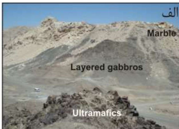
شکل ۲ رخنمون گابروهای لایه‌ای. الف- در مرز جنوبی، فرامافیک‌ها و در قسمت بالای گابروها مرمر رخنمون دارد، ب- لایه‌بندی تناوبی در گابروهای لایه‌ای.
