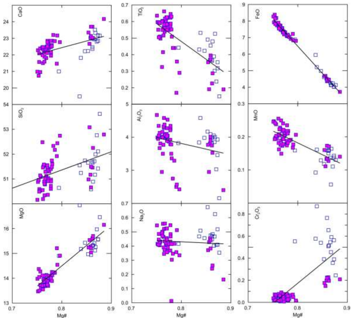
شکل ۶ نمودار تغییرات ترکیب کلینوپروکسن نسبت به Mg#.
