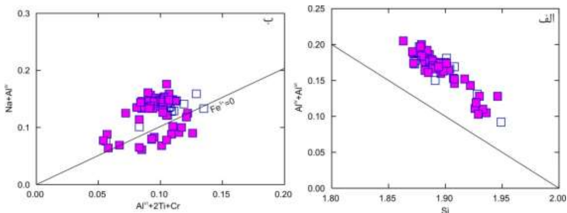
شکل ۸ الف- پیروکسن‌های مورد بررسی در نمودار Al نسبت به Si بالای خط اشباع جایگاه چاروچی قرار می‌گیرند [۳۱]. ب- قرار گیری نمونه‌های بالای خط Fe^{3+}=0 در نمودار Al^{VI}+2Ti+Cr نسبت به Na+Al^{IV} گویای گریزندگی بالای اکسیژن است [۳۱].
