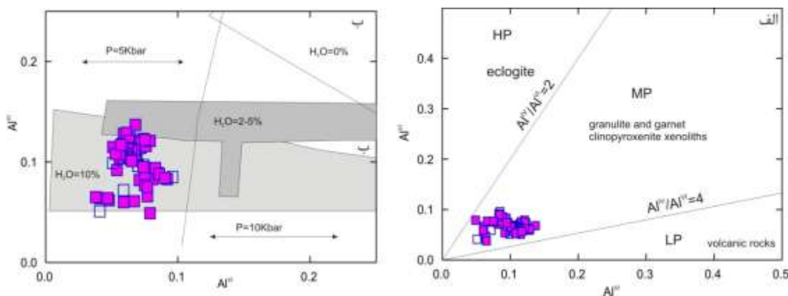
شکل ۹ الف- نمودار تغییرات Al^{VI} نسبت به Al^{IV} برای برآورد فشار تشکیل کلینوپیروکسن [۳۴]. (HP= میدان فشار بالا، MP= میدان فشار متوسط و LP=میدان فشار پایین). ب- نمودار توزیع آلومینیوم در جایگاه چاروچی و هشت وجهی، مقدار آب ماگما هنگام تبلور در حدود ۱۰٪ و فشار محیط تبلور کمتر از ۵ کیلو بار است [۳۷].
