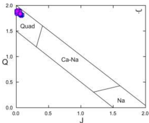
شکل ۴ موقعیت کلینوپیروکسن‌های گابروهای لایه‌ای جنوب ارزوتیه الف- در نمودار En-Fs-Wo [۱۶] و ب- در نمودار J-Q [۱۶]. J=2Na و Q=Ca+Mg+Fe^{2+} .
