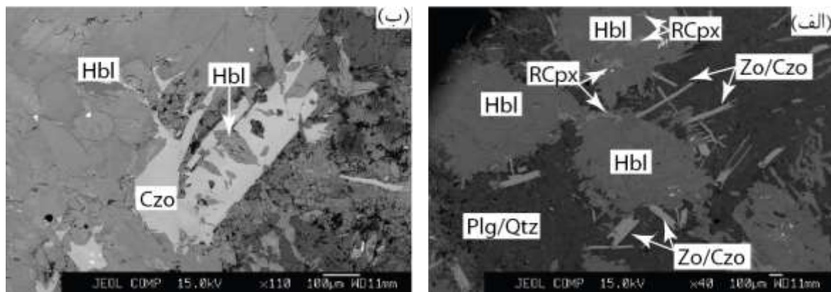
شکل ۳ تصاویر الکترون‌های پس پراکنده (BSE) از اپیدوت- آمفیبولیت‌های شمال ارومیه. (الف) منشورهای زوئیزیت و کلینوزوئیزیت به همراه هورنبلند، بقایای کلینوپیروکسن‌های اولیه در میان آمفیبول‌ها. (ب) بلورهایی از هورنبلند به صورت میانبار در کلینوزوئیزیت. Hbl: هورنبلند، Plg/Qtz: پلاژیوکلاز/ کوارتز، Zo/Czo: زوئیزیت/ کلینوزوئیزیت، Czo: کلینوزوئیزیت، RCpx: کلینوپیروکسن باقیمانده.
