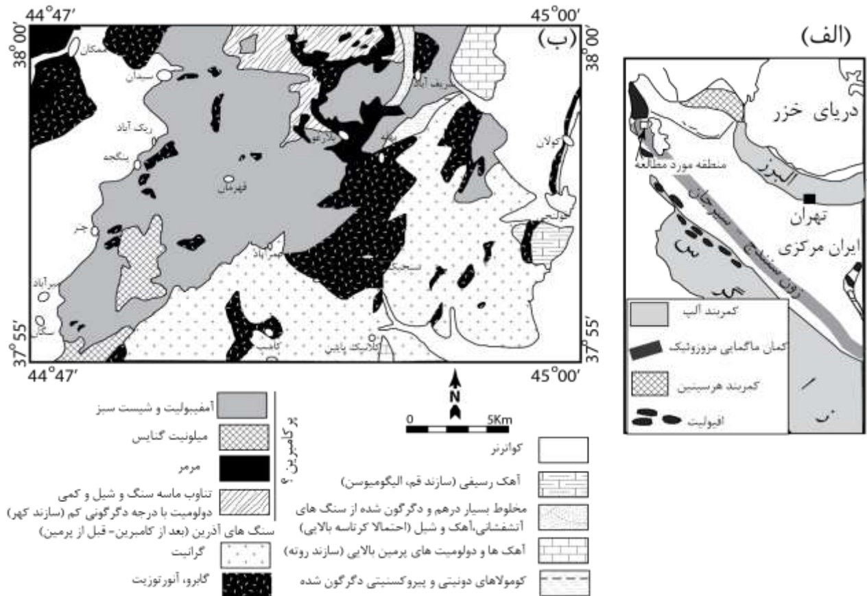
شکل ۱ (الف) موقعیت منطقه مورد بررسی در نقشه زمین‌ساختی ایران. برگرفته از مرجع [۱۴]. (ب) نقشه زمین‌شناسی ساده شده منطقه مورد بررسی. برگرفته از مرجع [۱۵].
