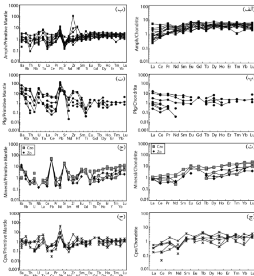
شکل ۴ الگوی عناصر خاکی نادر و نمودارهای چندعنصری برای کانی‌های آمفیبول، پلاژیوکلاز، کانی‌های گروه اپیدوت و کلینوپیروکسن‌های باقیمانده از سنگ اولیه.
