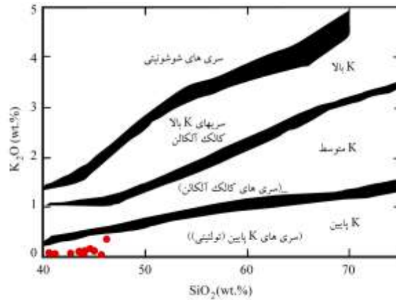
شکل ۵ تقسیم بندی سنگهای غیر آلکان با استفاده از نمودار K_2O در مقابل سیلیس [۵].
