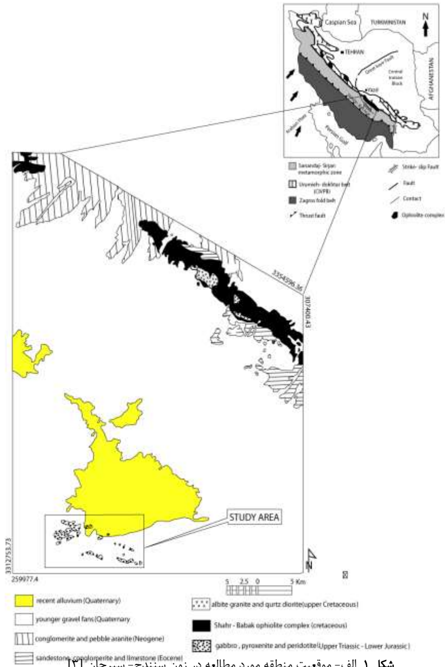
شکل ۱ الف- موقعیت منطقه مورد مطالعه در زون سنندج- سیرجان [۲]
