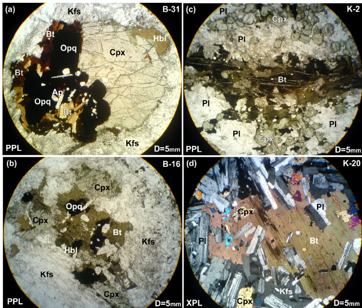
شکل ۲ تصاویر میکروسکوپی از بیوتیت نفلین سینیت بزقوش (a, b) و بیوتیت گابروی قلیایی کلیبر (c, d) و (a) بافت تجمعی که بواسطه حضور کانی‌های مافیک و کدر ایجاد شده است؛ (b) بیوتیت‌ها به طور مشخصی پیرامون کانی‌های کدر (اکسیدهای Fe-Ti) رشد کرده‌اند؛ (c) لامیناسیون (فولیاسیون) آذرین که بواسطه حضور بیوتیت ایجاد شده و (d) بیوتیت با بافت غربالی که دارای ورودی‌های پلاژیوکلاز، پیروکسن و اوپک است.
