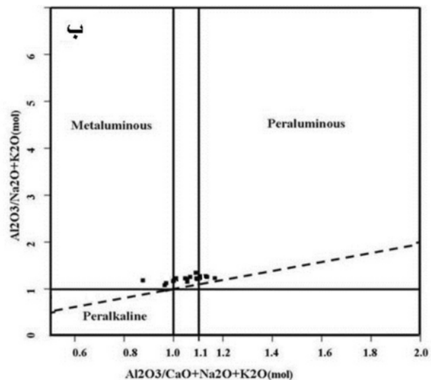
شکل ۵ الف) نمودار تغییرات Na_2O + K_2O نسبت به SiO_2 ، منحنی قلیایی، نیمه قلیایی اقتباس از [۴۷]. نمونه‌ها در گستره گرانیت قلیایی برجسته می‌شوند. ب) در نمودار شاخص اشباع شدگی از آلومینیم (ASI)، نمونه‌ها در گستره‌ی ۱-۱.۰ ASI = 1 با مقادیر بالای برای ضریب آگپانتی قرار می‌گیرند، ASI = 1.1 اقتباس از [۴۷] و ASI = 1.1 اقتباس از [۲۲]. نمودار بر اساس نسبت مولی است.
