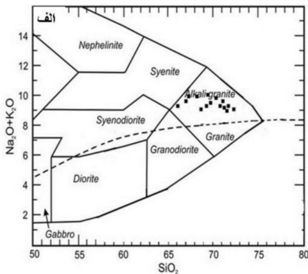
شکل ۵ الف) نمودار تغییرات Na_2O + K_2O نسبت به SiO_2 ، منحنی قلیایی، نیمه قلیایی اقتباس از [۴۷]. نمونه‌ها در گستره گرانیت قلیایی برجسته می‌شوند. ب) در نمودار شاخص اشباع شدگی از آلومینیم (ASI)، نمونه‌ها در گستره‌ی ۱-۱.۰ ASI = 1 با مقادیر بالای برای ضریب آگپانتی قرار می‌گیرند، ASI = 1.1 اقتباس از [۴۷] و ASI = 1.1 اقتباس از [۲۲]. نمودار بر اساس نسبت مولی است.
