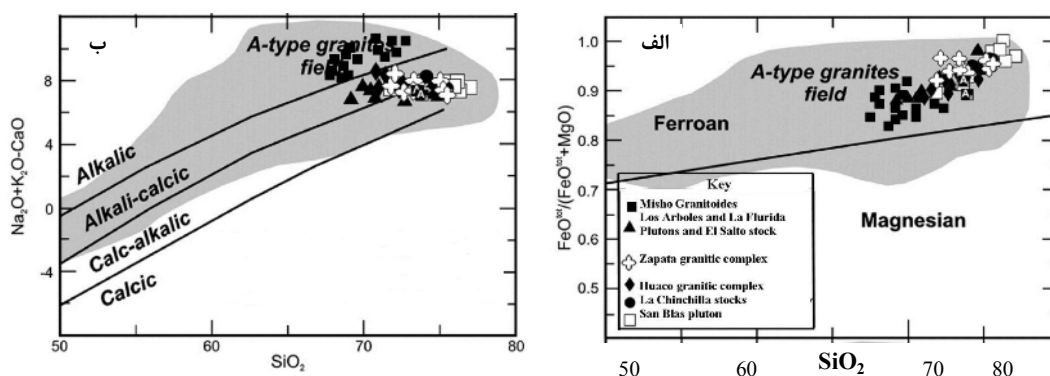
شکل ۶ الف) پلات گرانیت‌های مطالعه شده در دیگرام طبقه‌بندی FeO^3/(FeO^t + MgO) [۴۷] در مقابل SiO_2 (wt. % و ب) Na_2O + K_2O - CaO در مقابل SiO_2 نمونه‌ها در قلمرو گرانیت‌های نوع A آلکان قرار می‌گیرند. داده‌های شاهد اقتباس از [۲۰].
