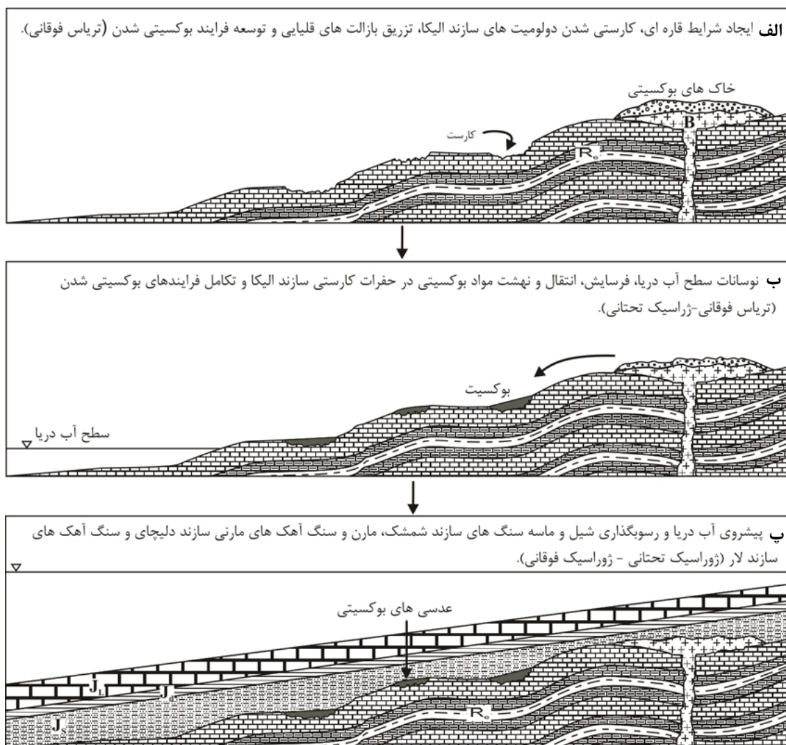
شکل ۸ مدل پیشنهادی برای تشکیل کنسار بوکسیت جاجرم. علامت‌های اختصاری به کار رفته عبارتند از: B= بازالت های قلیایی، R e = سنگ آهک مارنی، مارن و دولومیت‌های سازند الیکا، J= شیل و ماسه‌سنگ‌های سازند شمشک، J e = مارن و سنگ آهک‌های مارنی سازند دلیچای، J 1 = سنگ آهک‌های سازند لار.
