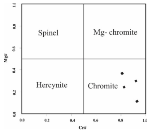
شکل ۷ موقعیت کرومیت‌های منطقه در نمودار Mg\#-Cr\# [۲۱].
