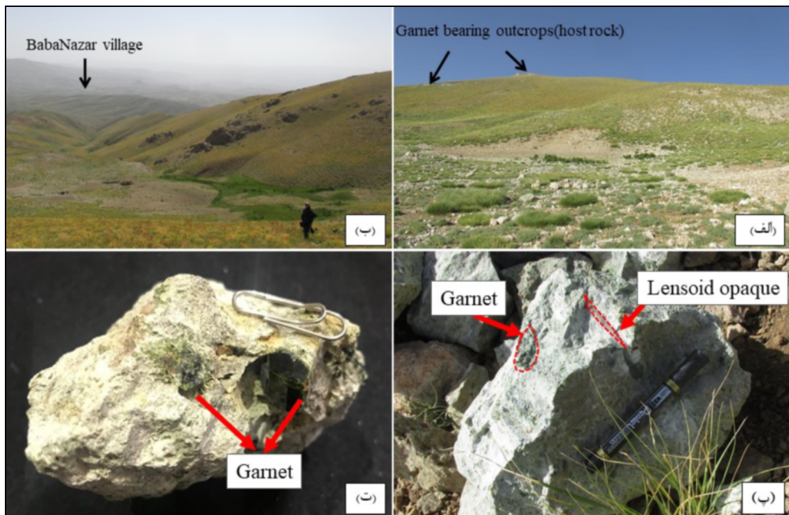
شکل ۲ الف- تصویر صحرایی از واحد گارنت یووارویت‌دار (دید به سمت شمال شرقی) ب- موقعیت رخنمون‌های گارنت‌دار (شاخص) نسبت به روستای بابانظر (دید به سمت جنوب غربی)، پ- نوارها و یا عدسی‌هایی از کانی کدر، ت- گارنت شکل دار به قطر ۲ سانتی‌متر و گارنت‌های بی‌شکل.
