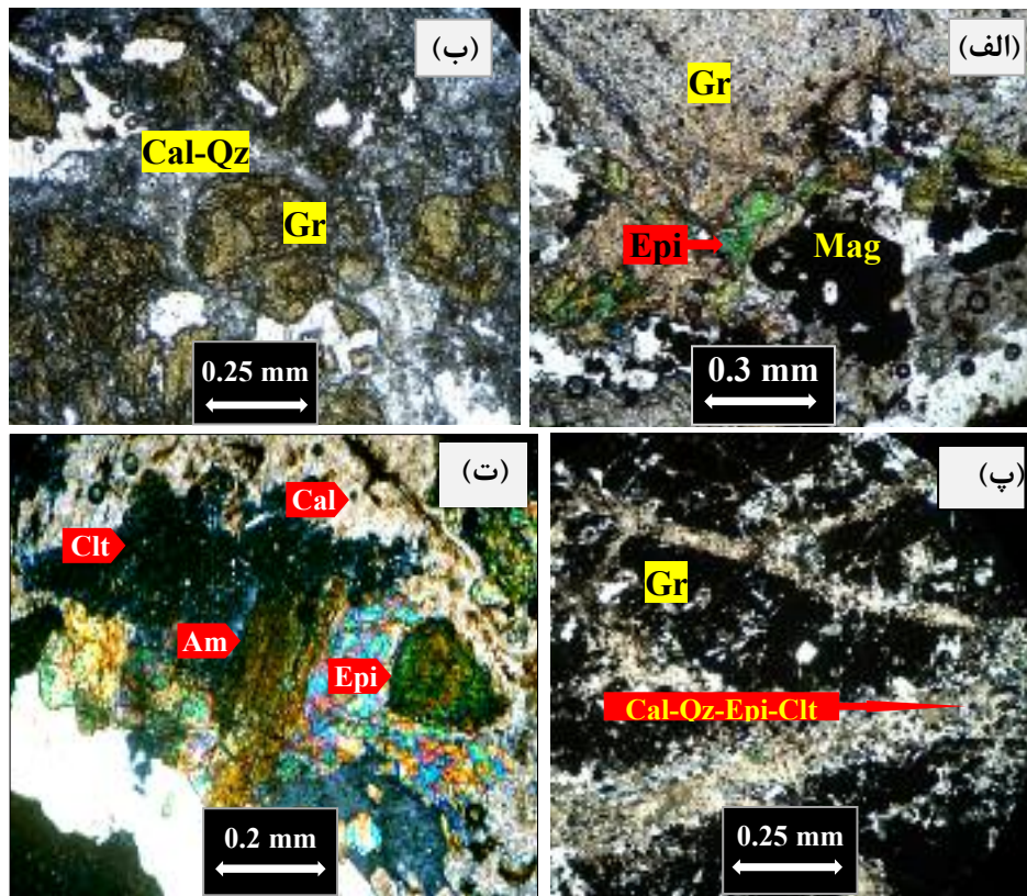
شکل ۴ (الف) تشکیل مگنتیت و اپیدوت از راه جانمایی گارنت (PPL)؛ (ب) خردشدگی و سیمانی شدن گارنت به وسیله کوارتز و کلسیت در مرحله دگرسانی قهقرایی (PPL)؛ (پ) قطع اسکارن پیشرونده با رگچه‌های اسکارن قهقرایی (XPL)؛ (ت) تشکیل کلریت از راه جانمایی اپیدوت و آمفیبول در مرحله دگرسانی پسرورنده (XPL)؛ (د) علایم اختصاری: Gr: گارنت، Mag: مگنتیت، Epi: اپیدوت، Cal: کلسیت، Qz: کوارتز، Clt: کلریت، Am: آمفیبول.
