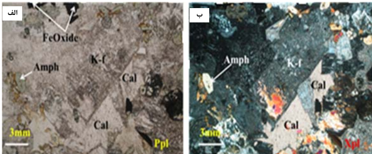
شکل ۴ تصویر یک نمونه مونزوسی‌نیت متشکل از ارتوزپریتی، پلاژیوکلاز، آمفیبول، اکسید آهن و کلسیت. کلسیت محصول دگرگانی است.
