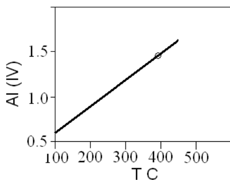
شکل ۶ محاسبهٔ دمای تشکیل کلریت براساس [۴]
