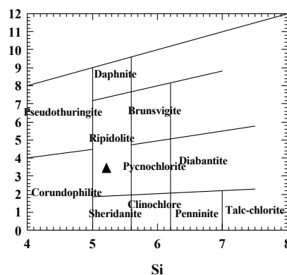
شکل ۵ ترکیب شیمیایی یک نمونه کلریت [۳].
