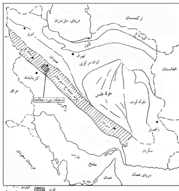
شکل ۱ موقعیت جغرافیایی زون سسندج-سیرجان، شهر همدان و رشته کوه الوند که منطقه مورد مطالعه بخشی از آن را شامل می‌شود.
