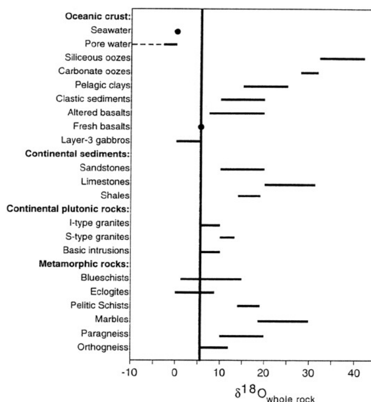
شکل ۷ نمودار مقادیر ایزوتوپی اکسیژن در سنگهای مختلف. در این نمودار مقادیر ایزوتوپی رگه‌های مورد مطالعه (۱۳ تا \delta^{18}\text{O} = 17\text{‰} در مقایسه با استاندارد SMOW) تقریباً مشابه مقادیر مربوط به شیستهای پلیتی است. اقتباس از [۲۵].
