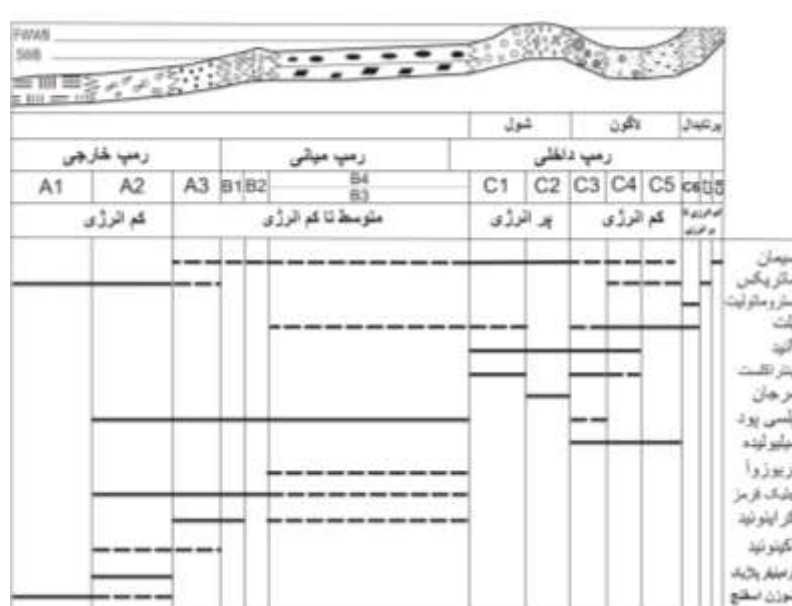
شکل ۱۱ طرحواره‌ای از محیط تهنشستی کربناته منطقه مورد مطالعه و تغییرات جانبی رخساره‌ها. در این طرحواره دانه‌های موجود با خط منقطع و دانه‌های فراوان با خط ممتد در هر رخساره مشخص شده است. حروف لاتین رخساره‌ها را نشان می‌دهد.
