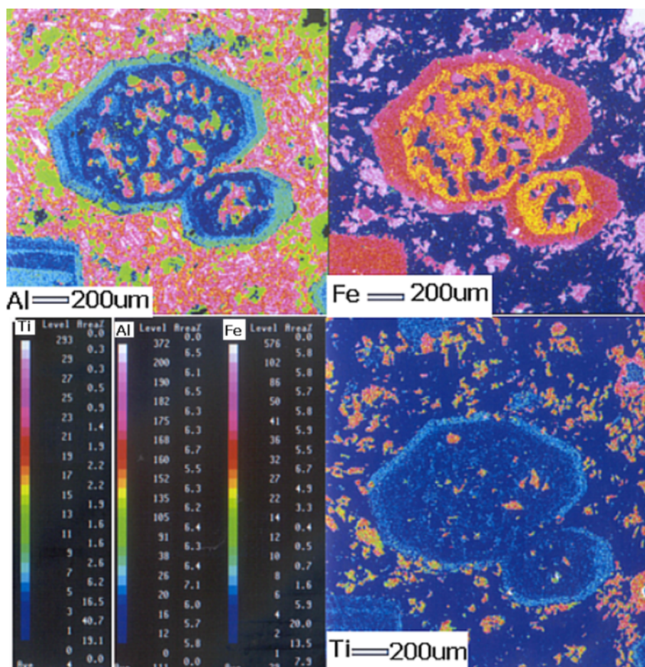
شکل ۴ نقشه توزیع عنصری از فنوکریست اسفنجی دیوپسید موجود در گدازه مؤزه آریتی که با ریزپدازنده الکترون تهیه شده است. چنانکه دیده می‌شود، میزان آلومینیم، تیتانیوم و آهن از مرکز به حاشیه افزایش می‌یابد.
