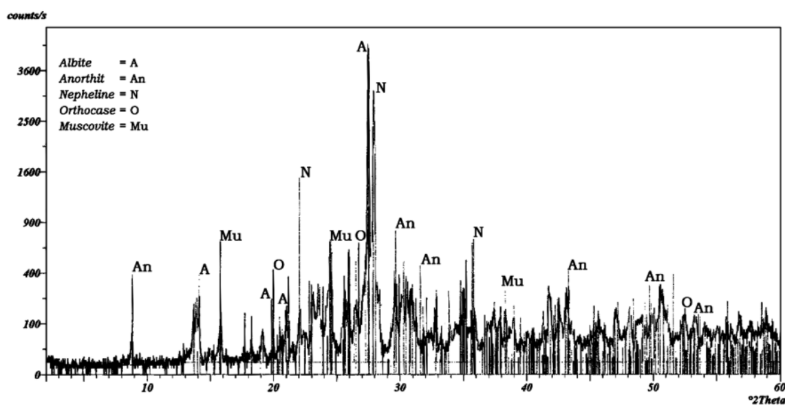
شکل ۱ آنالیز فازی (XRD) شیرۀ نفلین سینیت کلیبر.
