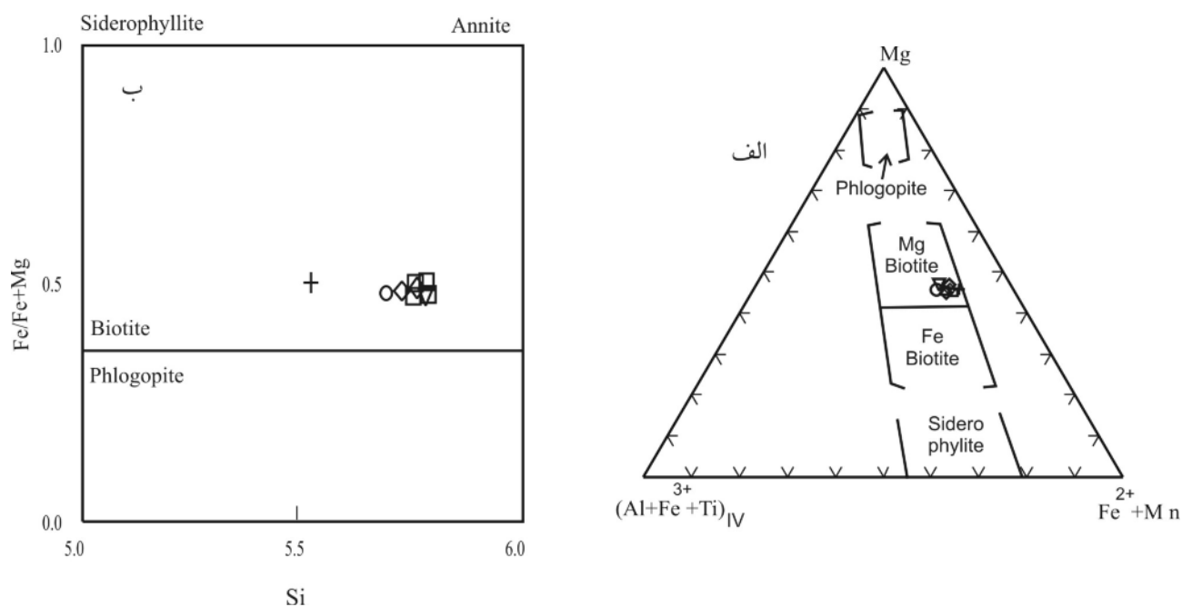
شکل ۲ طبقه‌بندی میکاها با استفاده از ترکیب شیمیایی آن‌ها (الف) فورستر، [۵] (ب) ریدر، [۶]. مربع نشان دهنده حاشیه بیوتیت در گرانودیوریت‌ها، لوزی معرف مرکز آن و علامت به علاوه نقطه‌ای بین حاشیه و مرکز است. مثلث نماینده حاشیه بیوتیت در دیوریت‌ها و دایره حاشیه آن را نشان می‌دهد.
