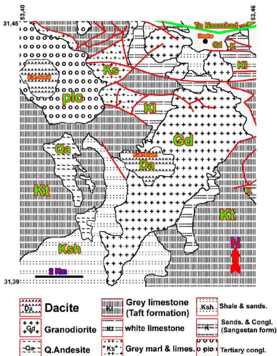
شکل ۱ نقشه زمین شناسی منطقه خوش (با تغییرات از [۴]).
