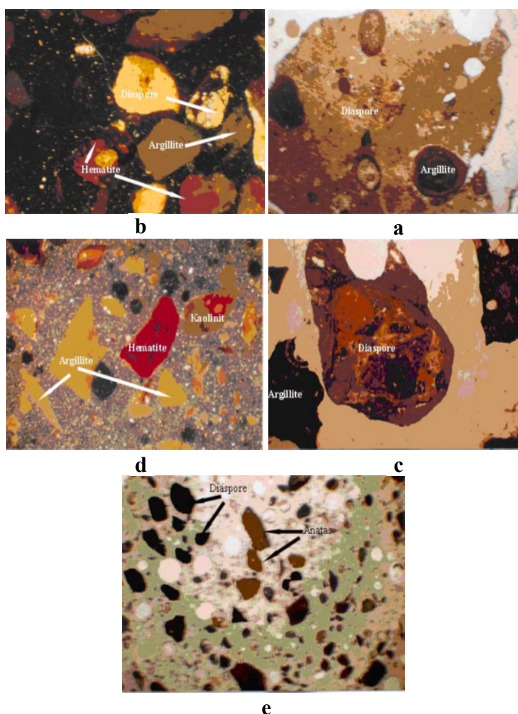
لوح ۱: تصاویر میکروسکوپی مقاطع نازک، نمونه‌ای از بافت‌ها و کانی‌ها در کانسار دویلان (۱۰۰×).
