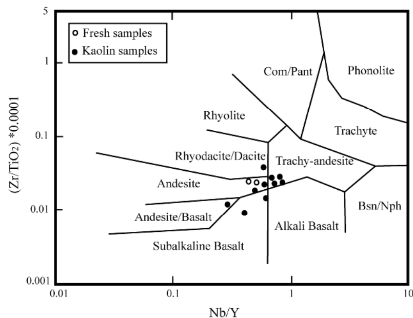
شکل ۵ موقعیت نمونه‌های وابسته به ذخیره‌ی کائولن هیزه‌جان و سنگ‌های آتشفشانی وابسته در نمودار دو متغیره‌ی \text{Nb/Y} - \text{Zr/TiO}_2 [۱۹].
