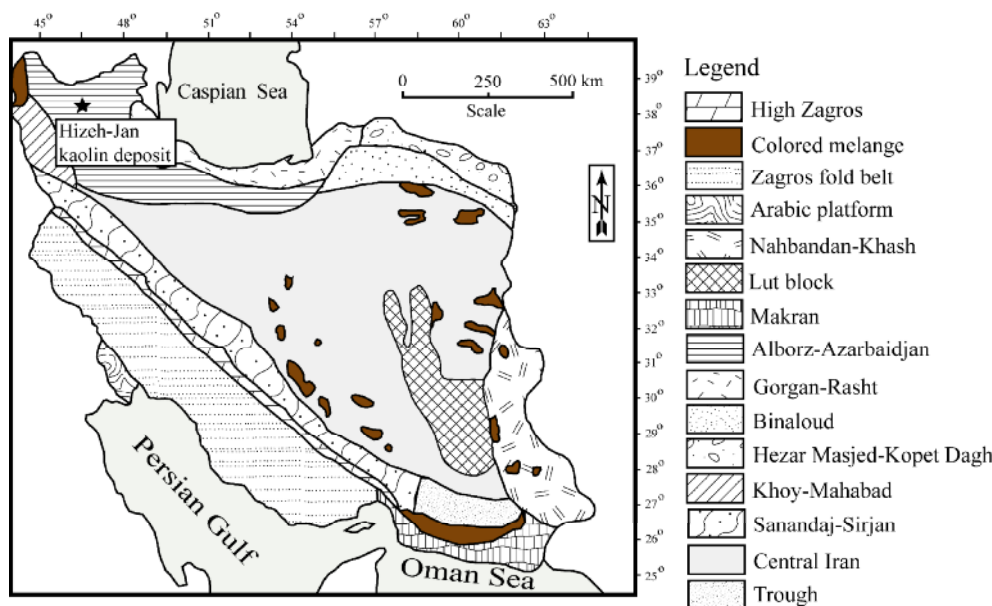
شکل ۱ نقشه‌ی پهنه‌های ساختاری ایران [۱۵] که بر اساس آن ذخیره کائولن هیزه‌جان در پهنه‌ی البرز- آذربایجان قرار می‌گیرد.
