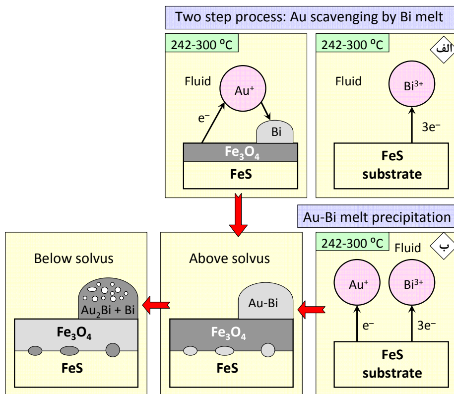
شکل ۹. مدل‌های نموداری تشکیل مذاب طلا-بیسموت (با تغییرات از [۲۱]). الف و ب) مدل اول: تشکیل غیرهمزمان یون‌های طلا و بیسموت در شارهی گرمایی و جدایش یون طلا به وسیله‌ی فاز آبگون بیسموتی با افزایش گریزندگی اکسیژن و نهشت آن در فضای خالی مگنتیت، پ، ت و ث) مدل دوم: تشکیل همزمان یون‌های بیسموت و طلا در سیال و احیاء آنها به وسیله پیرویت طی دو مرحله بالای سولوس و زیر منحنی سولوس. با توجه به عدم مشاهده پیرویت در منطقه، احتمالاً مدل نخست با شرایط کانی‌سازی منطقه کوه‌دم نزدیکتر است.
