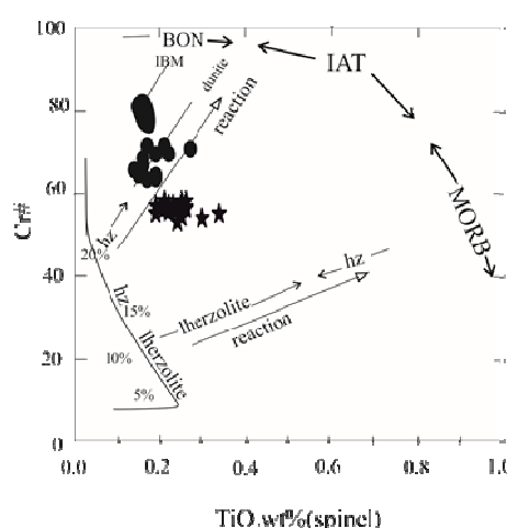
شکل ۷ تغییرات Cr# در مقابل \text{TiO}_2 ، اسپینل‌های دونیت‌های پیوسته و دایک‌های دونیتی در دو گستره‌ی مجزا قرار می‌گیرند. (FMM = گوشته مورب بارور، IBM = ایزوبونین ماریانا، IAT = تولئیت‌های جزایر قوسی، IBM = بونینیت) [۱۴، ۱۵].
