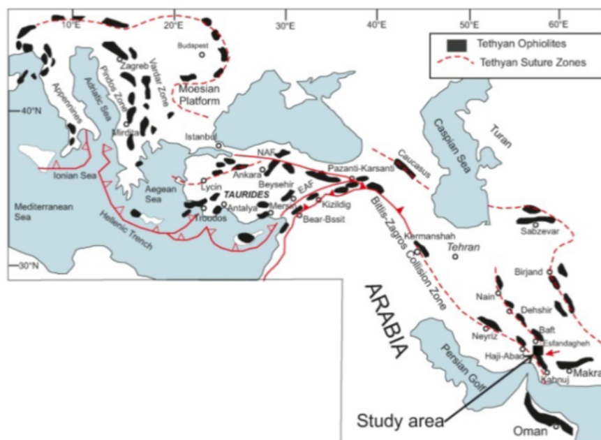
شکل ۱ بخشی از کمر بند کوهزایی آلپ - هیمالیا (افیولیت‌های تتیسی) به همراه با موقعیت افیولیت‌های ایران و منطقه‌ی مورد بررسی [۷].
