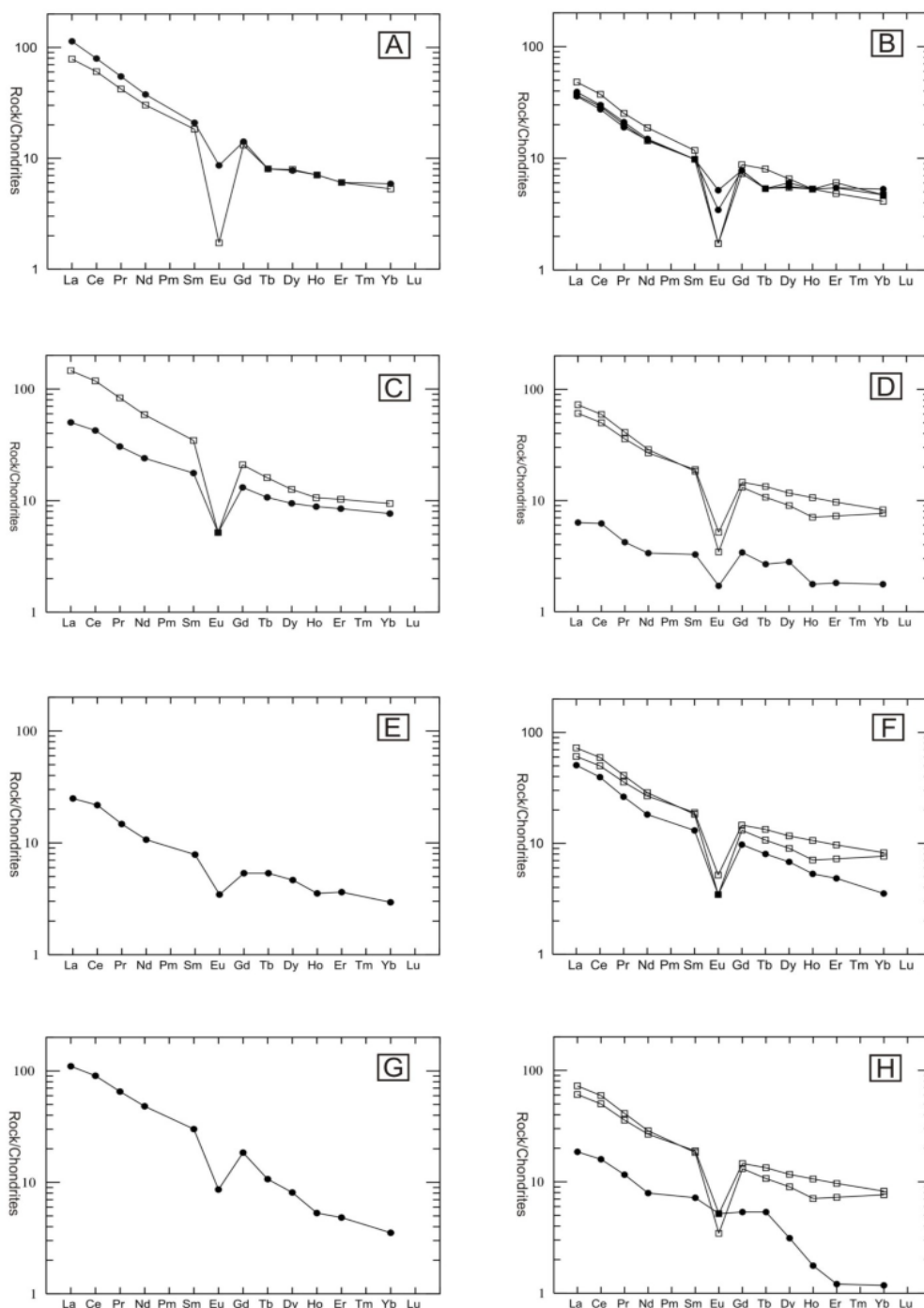
شکل ۷ نمودار بهنجارشده نسبت به کندریت برای نمونه‌های منطقه مورد مطالعه با استفاده از داده‌های [۲۵]: (A) زون سریسیتی؛ (B) زون کلریتی؛ (C) زون پروپیلیتی؛ (D) زون آرژیلیتی؛ (E) زون سیلیسی؛ (F) زون آلبیتی؛ (G) زون هماتی؛ (H) زون تورمالینی. • نمونه دگرسان شده، □ نمونه دگرسان نشده.
