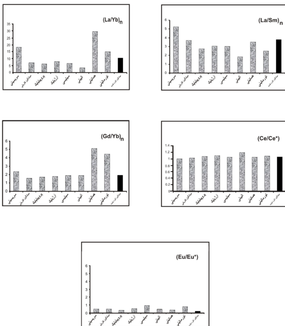
شکل ۸ نسبت‌های (La/Yb)_n , (Gd/Yb)_n , (Ce/Ce^*) و (Eu/Eu^*) وابسته به زون‌های مختلف دگرسان منطقه آستانه در مقایسه با میانگین نمونه‌های دگرسان نشده.
