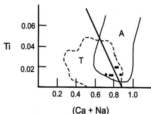
شکل ۱۱ نمودار جدایش فنوکریست‌های کلینوپیروکسن در بازالت‌ها [۲۷]. نمودار Ti نسبت به (Ca+Na) که گستره بازالت‌های تولئیتی (T) و دیگر بازالت‌ها (A) را از یکدیگر جدا می‌کند.
