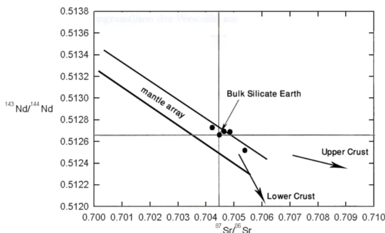
شکل ۱۸ موقعیت بازالت‌های جواهردشت در نمودار همبستگی ایزوتوپی \text{Nd}-\text{Sr} . روند پسته فوقانی و تحتانی از یونگ [۲] اقتباس شده است.
