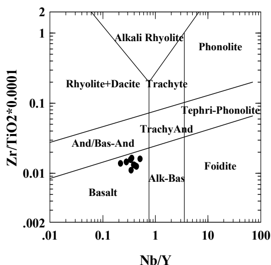
شکل ۸ موقعیت نمونه‌ها در نمودار وینچستر و فلوید [۵].
