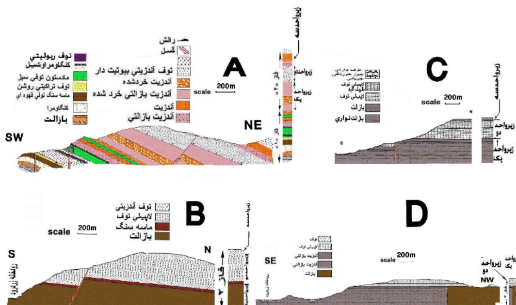
شکل ۲ الف) مقاطع زمین‌شناسی و ستون‌های چینه‌شناسی فاز دوی پالوژن وابسته به (A) باختر تنگه‌رود، (B) یک کیلومتری خاور زرد رود، (C) جنوب گلک، (D) جنوب کارخانه سیمان، (E) جنوب خاوری گرم‌اور، (F) جنوب لرو، (ب) تغییرات ضخامت و جنس دنباله زیرواحدهای فاز دو در طول منطقه مورد بررسی از باختر به خاور (برای تشخیص علائم و نشانه‌های به کار رفته به راهنماهای شکل ۲-الف مراجعه کنید).
