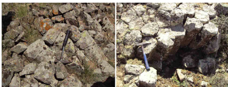
شکل ۶ ساخت منشوری در بازالت‌های وابسته به فاز دوی پالئوژن منطقه مورد بررسی.
