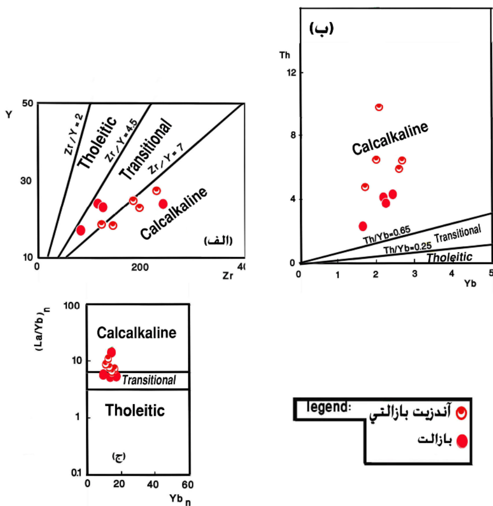
شکل ۱۰ داده‌های وابسته به سنگ‌های آتشفشانی فاز دوی پالئوژن روی نمودارهای الف) Y-Zr، ب) Th-Yb، ج) La_N/Yb_N - Yb_N .
