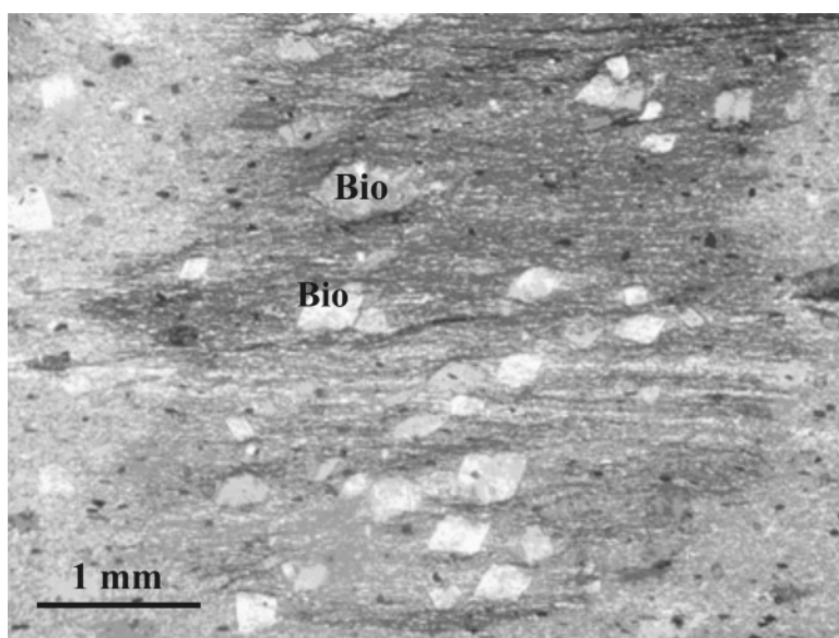
شکل ۱ پورفیروبلاست‌های بیوتیت (Bio) در زون بیوتیت. به چرخش شیسستوزیته در پیرامون بیوتیت‌ها توجه کنید.
