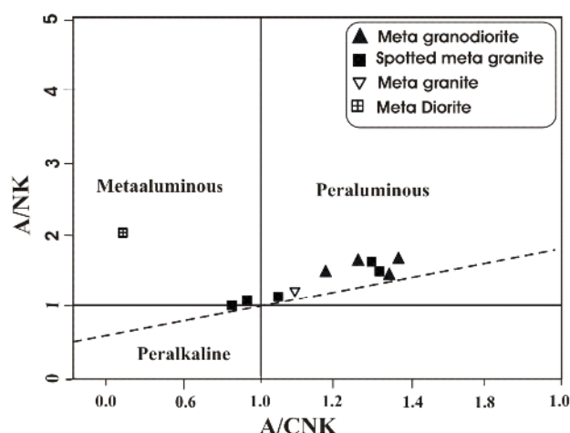
شکل ۶ نمودار تعیین میزان Al توده‌های اواسط - اواخر پالئوزوئیک [۱۳].
