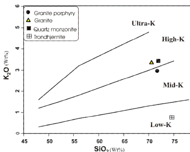
شکل ۱۲ نمودار تعیین میزان پتاسیم [۱۲].
