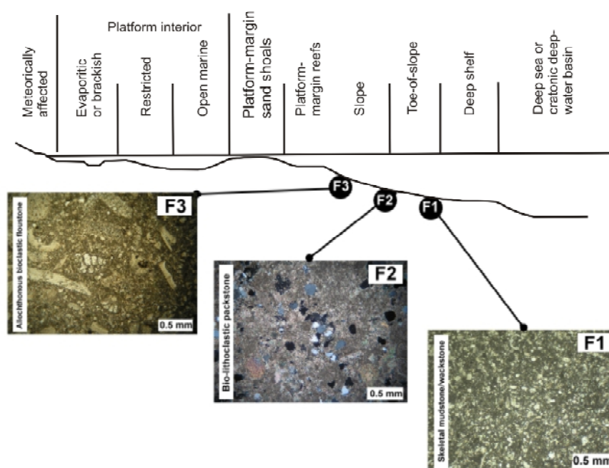
شکل ۵ موقعیت نسبی رخساره‌های F1، F2 و F3 در طاقچه کربناته که در قیاس با رخساره‌های استاندارد [۹]، نمایش داده شده‌اند. چنانچه که مشاهده می‌شود تنوع رخساره‌ای این دنباله بسیار پایین بوده و در کل رخساره‌های نواحی نسبتاً عمیق اقیانوسی را نشان می‌دهند.
