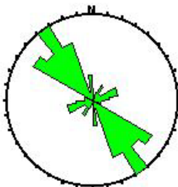
شکل ۲ نمودار گل سرخی وابسته به شکستگی‌های کانی‌زایی شده در گستره‌ی مورد بررسی. شکستگی‌های با روند شمال باختری - جنوب خاوری میزبان رگه‌های معدنی است که خود در اثر شکستگی‌های با روند کلی خاوری باختری قطع شده‌اند.
