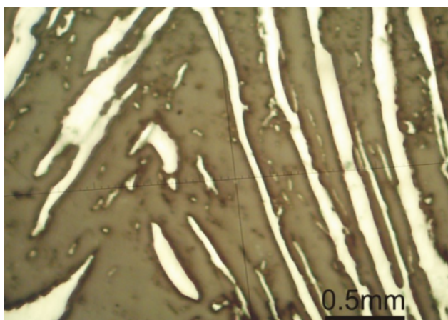
شکل ۴ بافت زین‌اسبی در استینیت‌های رگه شماره ۲ در برش صیقلی در PPL. رگه‌های استینیت با رنگ سفید مایل به خاکستری در بستر باطله سیلیسی قرار دارد.
