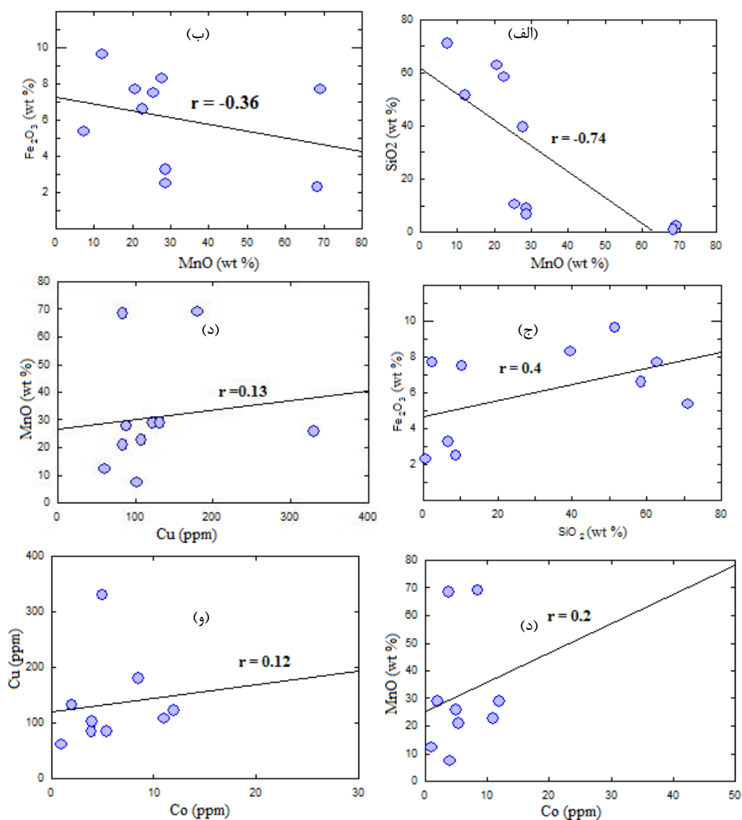
شکل ۸ نمودارهای همبستگی به‌ترتیب MnO نسبت به SiO 2 و Fe 2 O 3 (الف و ب)، SiO 2 نسبت به Fe 2 O 3 (ج)، MnO نسبت به Co و Ni (د) و Cu نسبت به Co (و)، و Cu نسبت به Co (و).
