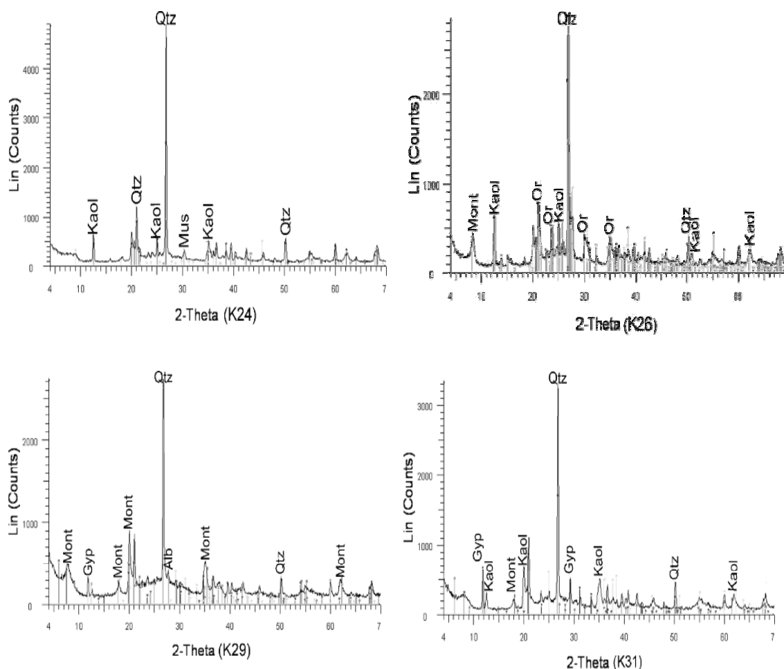
Qtz: کوارتز Mont: مونتموریونیت Kaol: کائولینیت Mus: مسکویت Gyp: ژپس Alb: آلبیت Or: اورتوکلاز شکل ۴ تصاویر ۴ نمونه از قله‌های XRD کائولینیت‌های شیخ آباد.
