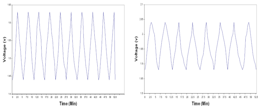
شکل ۴ نمودار ولتاژ-زمان بلور \text{K}_{1-x}(\text{NH}_4)_x\text{H}_2\text{PO}_4 با x = ۰٫۱ مربوط به وجه (الف) [۱۰۰] و (ب) [۱۰۱].
