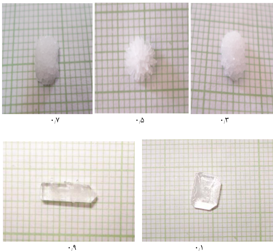
شکل ۳ بلورهای \text{K}_{1-x}(\text{NH}_4)_x\text{H}_2\text{PO}_4 با مقادیر ۰٫۹، ۰٫۷، ۰٫۵، ۰٫۳، ۰٫۱ و x = ۰٫۱
