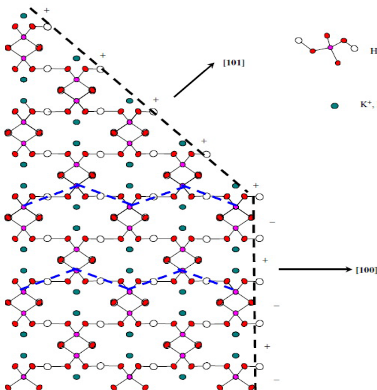
شکل ۱ طرح وارهای آرایش اتمی سطوح (۱۰۰) و (۱۰۱) بلورهای خانواده KDP [۱۲].
