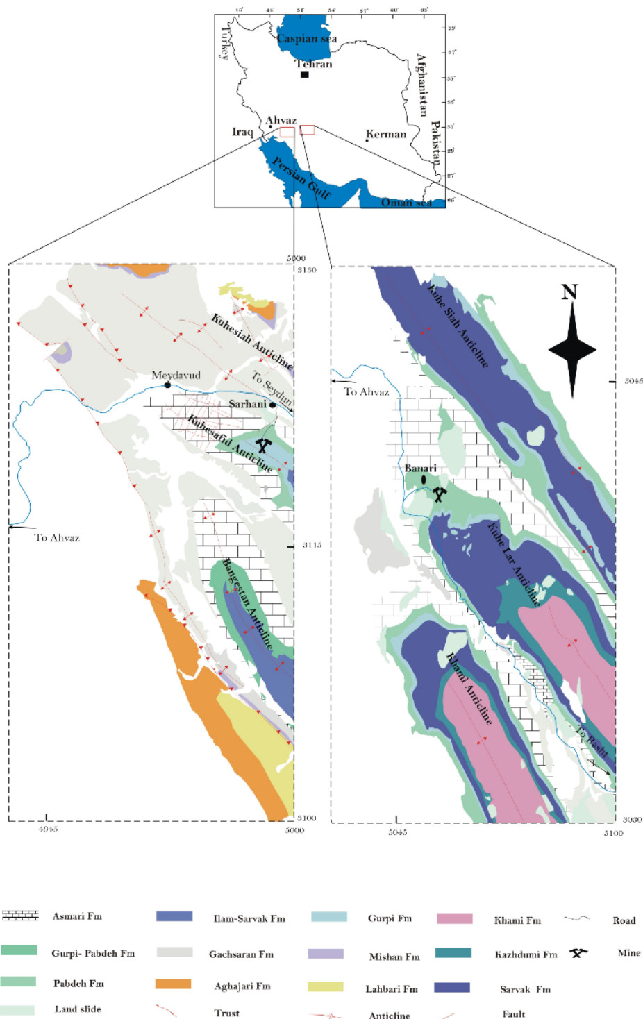
شکل ۱ نقشه‌ی زمین‌شناسی (برگرفته از نقشه‌های یک صد هزار کوه سفید و دهدشت، ترسیم شده به وسیله‌ی شرکت نفت) و موقعیت جغرافیایی مناطق مورد بررسی (مقیاس: ۱:۶۰۰۰).
