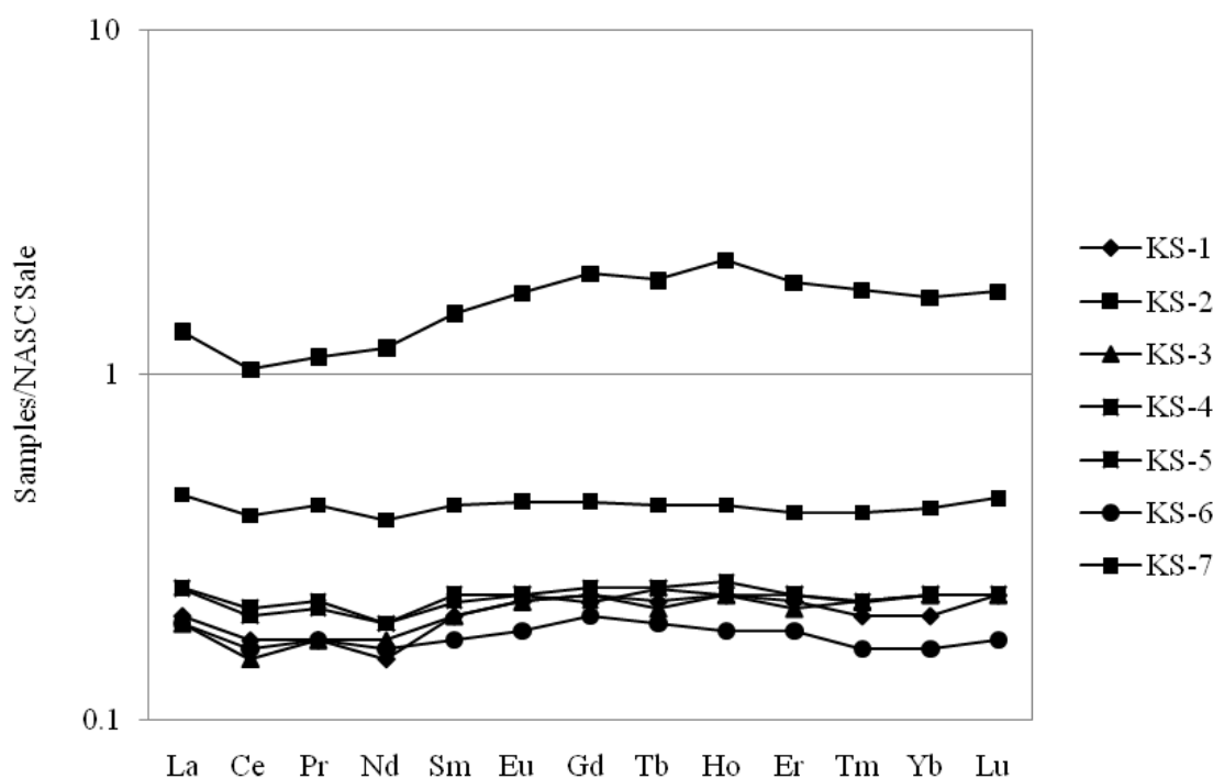
شکل ۶ الگوی تغییرات REE بهنجار شده نسبت به NASC [۱۷] کانسار فسفات کوه سفید.
