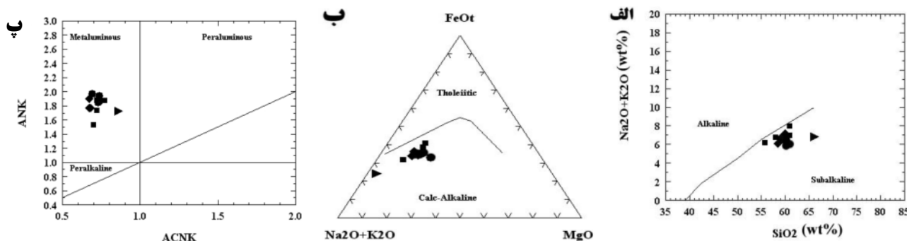
شکل ۴ (الف) نمودار مجموعه‌ی Na_2O + K_2O نسبت به SiO_2 برای تمایز سری‌های قلیایی از شبه قلیایی [۲۶]؛ (ب) نمودار مثلثی AFM [۲۶]؛ (پ) نمودار ANK نسبت به ACNK [۲۷]. نشانه‌ها بر اساس شکل (۳) است.
