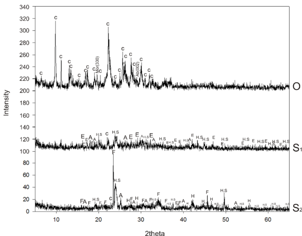
شکل ۶ نمودارهای پراش پرتو ایکس نمونه‌ی اولیه (O)، نمونه‌ی سنتزی ( S_{1b} )، و نمونه‌ی سنتزی دوم ( S_{2b} )، در نمودارهای مورد نظر، (C) : کلینوبیتولیت، (Mor) : مور دنت، (Ab) : آل بیت، (E) : ادینگتونیت، (H) : هارموتوم، (F) : فوجاسیت، (A) : آنالسیم و (H.S) : هیدروسودالیت.
